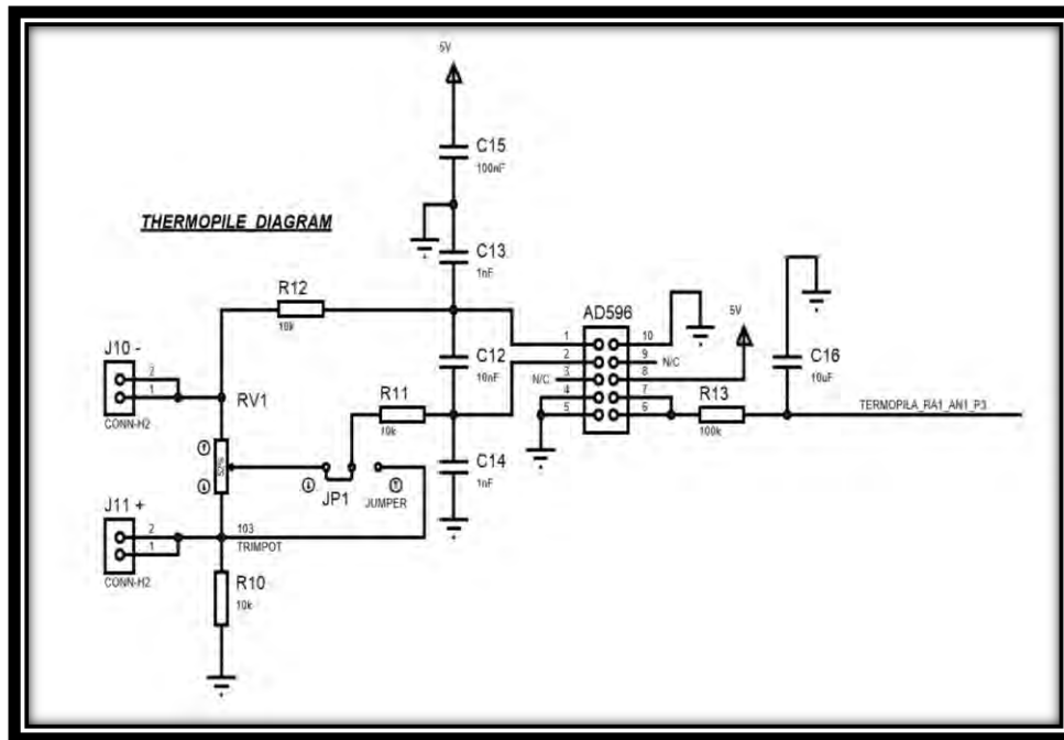
Figura 2. Diagrama final de conexión del termopar.
