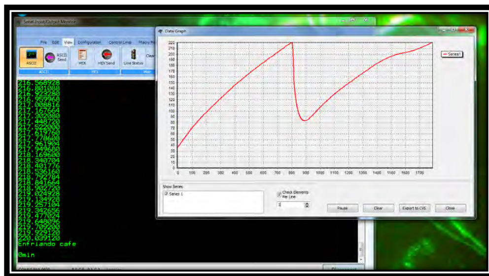
Figura 3. Prueba de medición de curvas de temperaturas del café.
