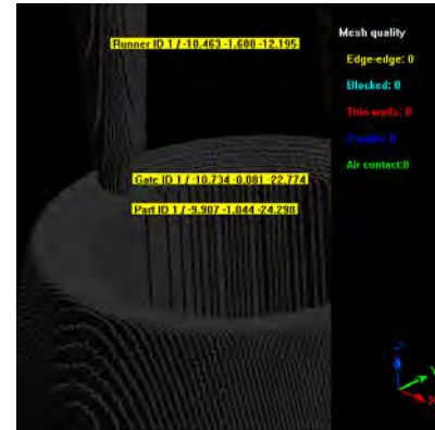
Figura 8. Reporte de la calidad del mallado.
