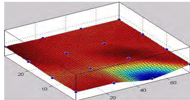
Gráfica 4. Distribución espacial de la lluvia simulada durante 20 ms de apertura de la electroválvula.
