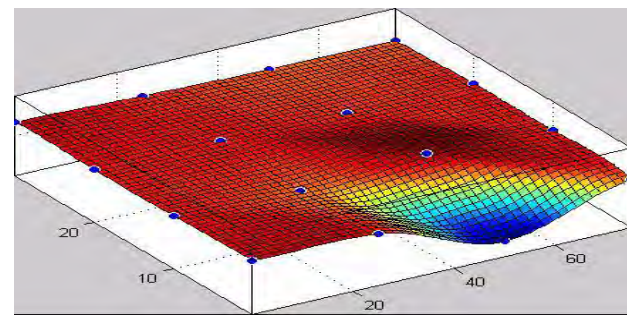
Gráfica 6. Distribución espacial de la lluvia simulada durante 40 ms de apertura de la electroválvula.
