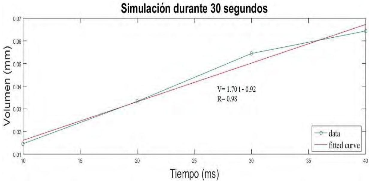
Gráfica 2. Comportamiento del volumen de agua con base a la curva de ajuste realizada y su ecuación lineal.
