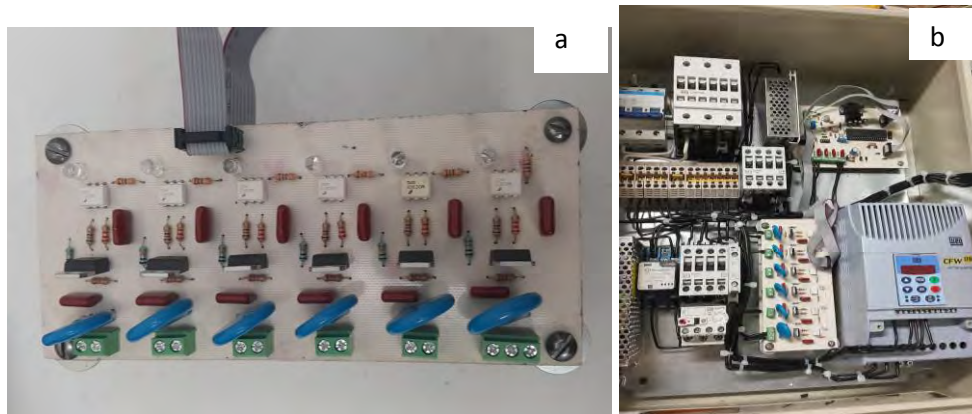
Figura 4. a.-Tarjeta de potencia finalizada; b.-Platina de control
