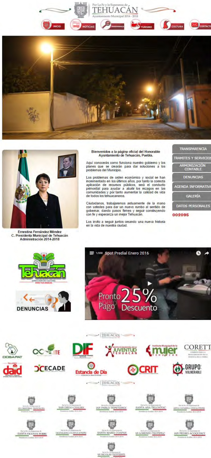
Figura 2. Página web 2015
