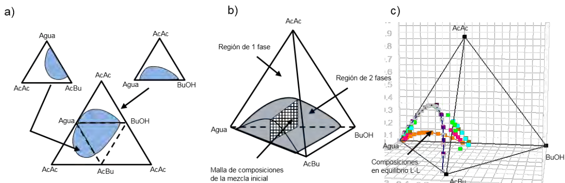
Figura 1. Determinación cualitativa y cuantitativa del equilibrio líquido-líquido. a) Distribución y representación de las curvas de solubilidad, b) malla de composiciones globales iniciales de la mezcla y c) Composiciones en equilibrio líquido-líquido.
