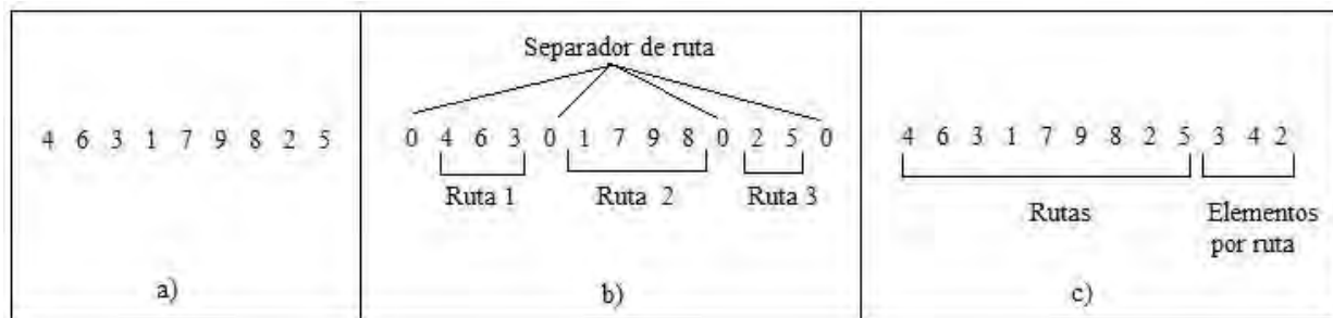
Figura 2. Ejemplo de las representaciones para ruteo de vehículos.
