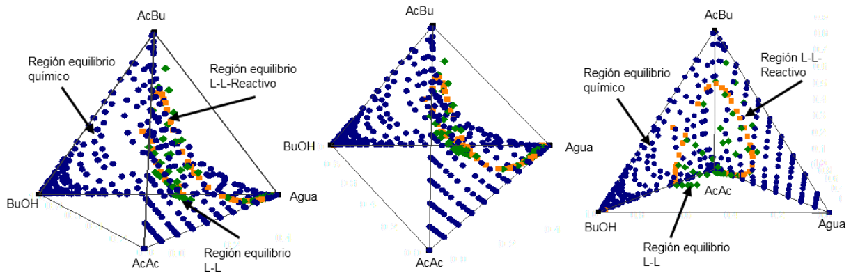
Figura 4. Diversas proyecciones de los equilibrios termodinámicos. La región con puntos azules representa el equilibrio químico, la de puntos verdes corresponde al equilibrio líquido-líquido y la de puntos naranjas al equilibrio líquido-líquido reactivo.
