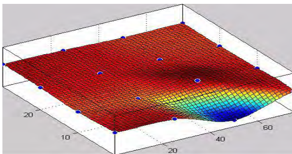
Gráfica 5. Distribución espacial de la lluvia simulada durante 30 ms de apertura de la electroválvula.
