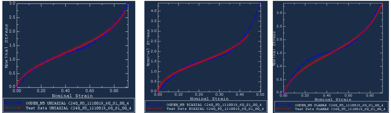
Figura 3. Ajuste de los datos experimentales con teoría Ogden de 5º orden.
