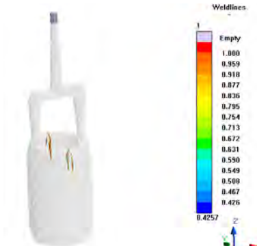
Figura 12. Líneas de soldadura del hule.
