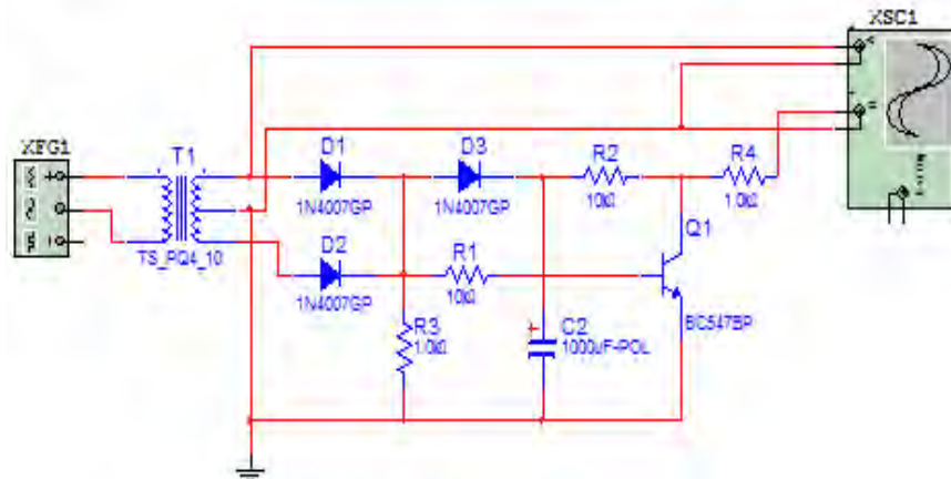
Figura 2. Diagrama eléctrico de los componentes para el control de la electroválvula.
