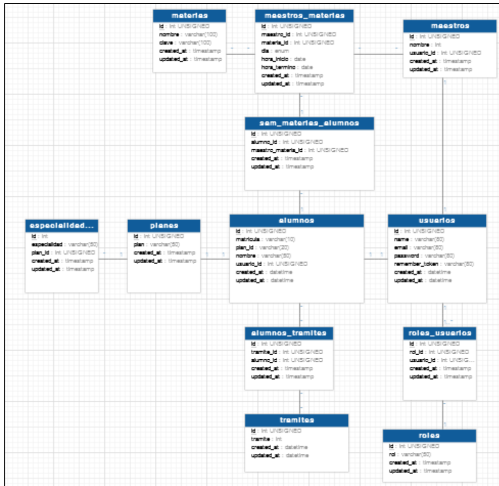
Figura 2. Modelo Relacional de Base de Datos simplificado del programa.
