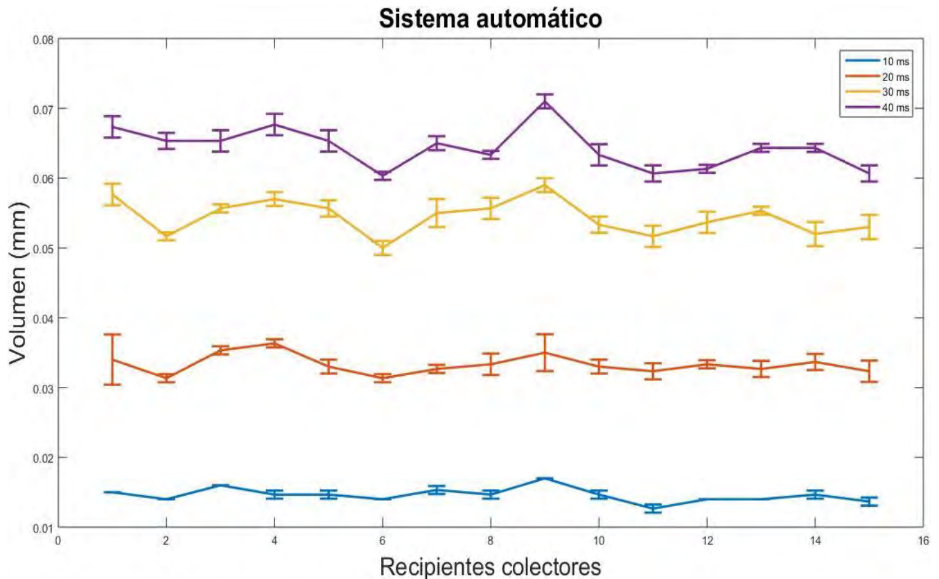
Gráfica 1. Distribución del comportamiento del volumen de agua acumulado durante los diferentes tiempos de experimentación.
