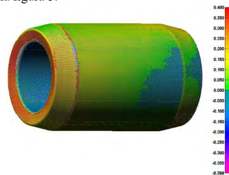
Figura 6. Mapa de desviación que muestra la diferencia entre el modelo CAD de la pieza esperada contra la real a temperatura ambiente de 24 °C.
