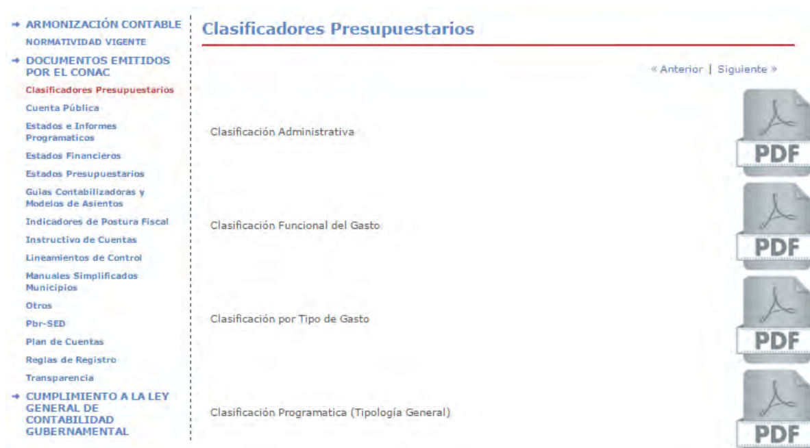
Figura 4. Armonización contable
