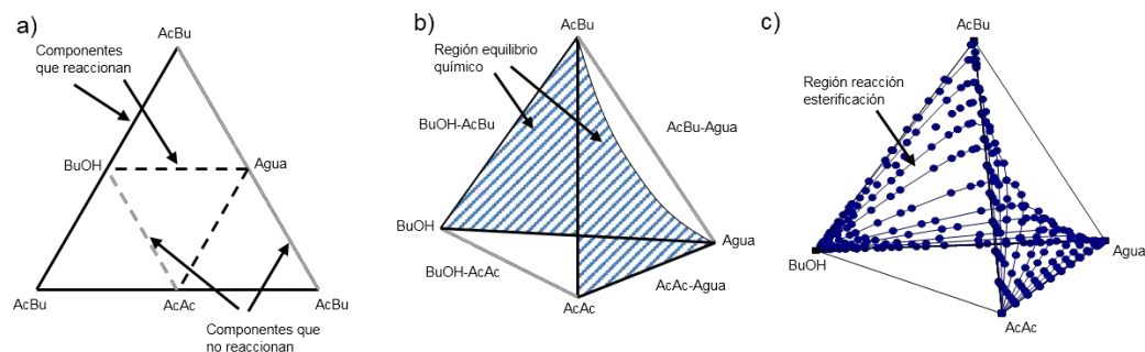
Figura 2. Determinación cualitativa y cuantitativa del equilibrio químico. a) Distribución y representación de los componentes reactivos y no reactivos, b) bosquejo del equilibrio químico y c) Composiciones en equilibrio químico.
