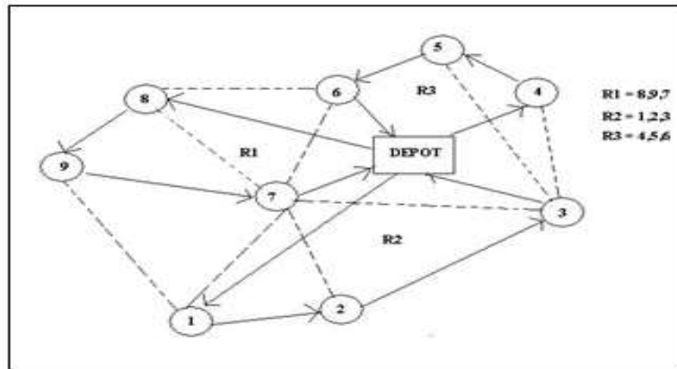
Figura 1. Ejemplo del CVRP para 9 clientes. Fuente: Elaboración propia.
