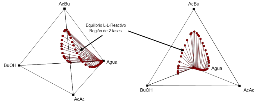
Figura 3. Perspectivas de las composiciones del equilibrio líquido-líquido reactivo. La región delimitada por puntos corresponde a la región de dos fases y las líneas representan líneas de reparto reactivas.
