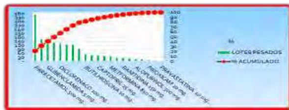
Gráfica 1 Diagrama de Pareto
