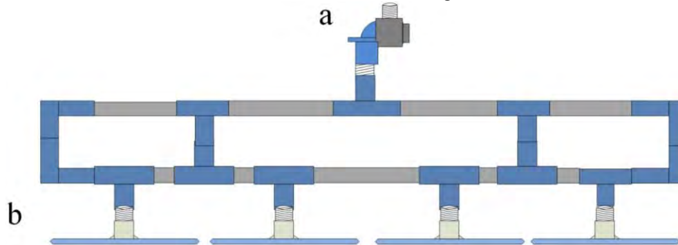
Figura 1. Diagrama de la distribución del sistema generador de gotas; a) electroválvula de 120 volts; b) Fila de regaderas cuadradas.
