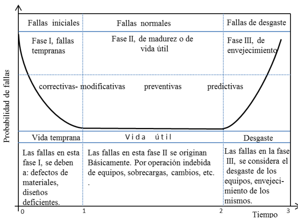
Figura 1 Curva de la bañera y acciones requeridas.
