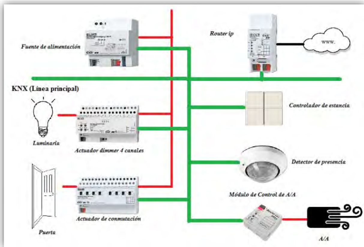
Figura 2. Esquema de la instalación propuesta en el modelo
