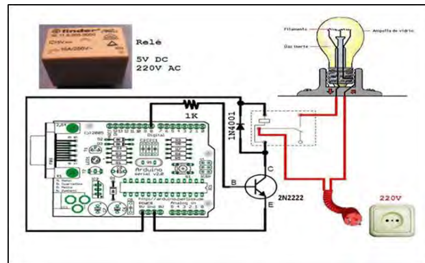
Figura 3. Esquema general del circuito eléctrico.
