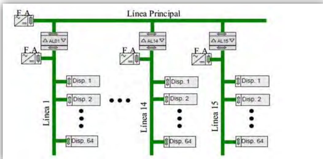
Figura 1. Esquema de un área en la topología EIB
