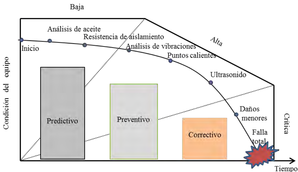
Figura 2. Identificación de defectos.
