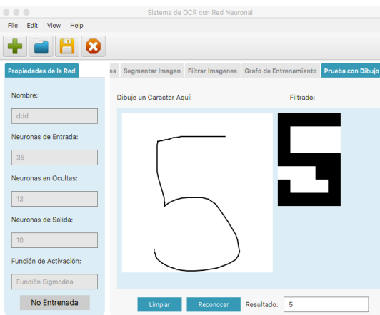
Figura 8. Reconocimiento de Dígito
