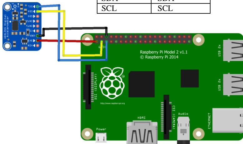
Figura 3. Conexión física entre el acelerómetro ADXL345 y la Raspberry Pi
