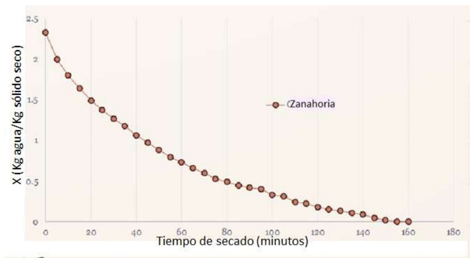
Figura 2. Curva de disminución de humedad de zanahoria con respecto al tiempo
