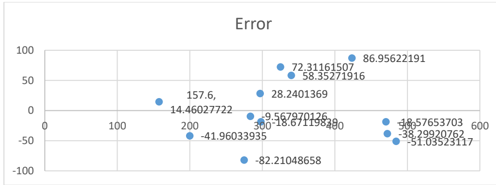
Figura 2. Gráfico de residuales
