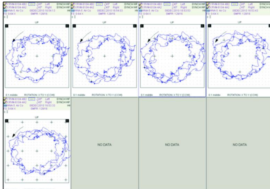
Figura 3.0 Estos gráficos de órbitas muestran la precesión errática del eje que existía cuando se estaba estableciendo la condición de látigo, solo unos minutos antes de que ocurriera el disparo de alta vibración.
