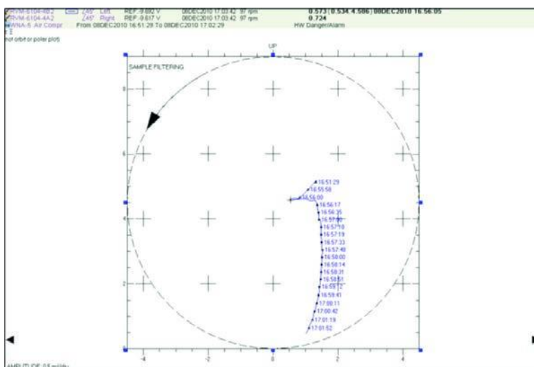
Figura 2.6 La posición media del rotor de la turbina de vapor parece moverse hacia una relación de excentricidad más baja (más cerca de la línea central del orificio del rodamiento) en el momento de la vibración elevada que provocó el disparo.
