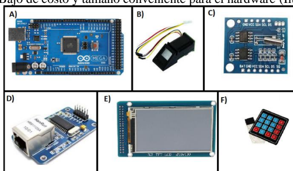
Ilustración 2 Componentes del sistema de reloj biométrico. A) Placa Arduino Mega 2560. B) Sensor de huellas dactilares (ER-SOT6439F) DSP AS601. C) Módulo tiny RTC (Real Time Clock). D) Módulo Ethernet Enc28j60. E) Módulo Display TFT LCD. F) Teclado Matricial 4x4.
