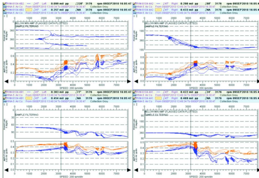
Figura 3.6 Prueba de solo turbina de la prueba de sobre velocidad de rutina de 09SEP2010, mostrando pequeñas amplitudes de vibración.
