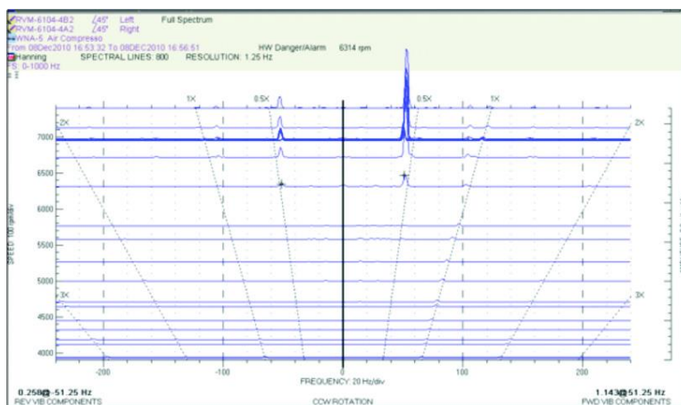
Figura 2.8 Diagramas en cascada para el disparo de la turbina y el evento de exceso de velocidad. La inestabilidad del rotor apareció por encima de 6314 RPM a una pequeña amplitud.
