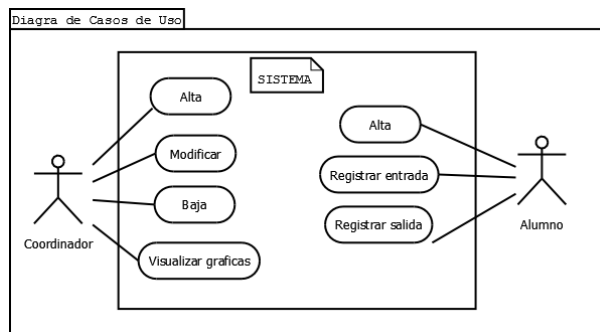
Ilustración 7 Diagrama de casos de uso de Samia.
