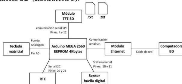
Ilustración 3 Diagrama general del sistema del reloj biométrico.
