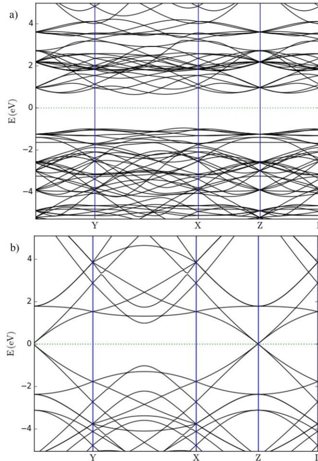
Figura 3. a) Estructura de bandas del cristal de WSe 2 , b) Estructura de bandas del grafeno.
