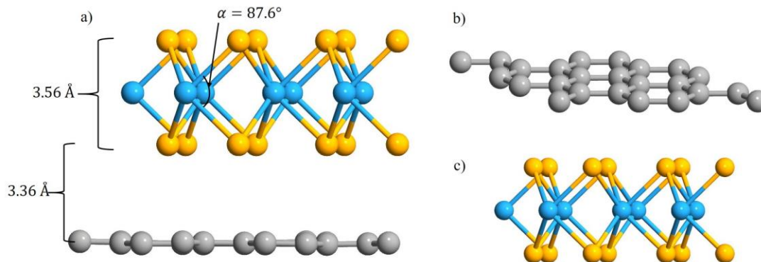
Figura 2. a) heteroestructura de Gr/ WSe_2 , b) hoja de grafeno y c) hoja de WSe_2 .
