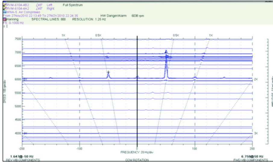
Figura 3.3 Para el evento 27NOV2010, la frecuencia de excitación también fue de aproximadamente 50 Hz. Observe que una fuerte precesión hacia delante apareció por primera vez al alcanzar los 6038 rpm a medida que aumentaba la velocidad de la máquina.
