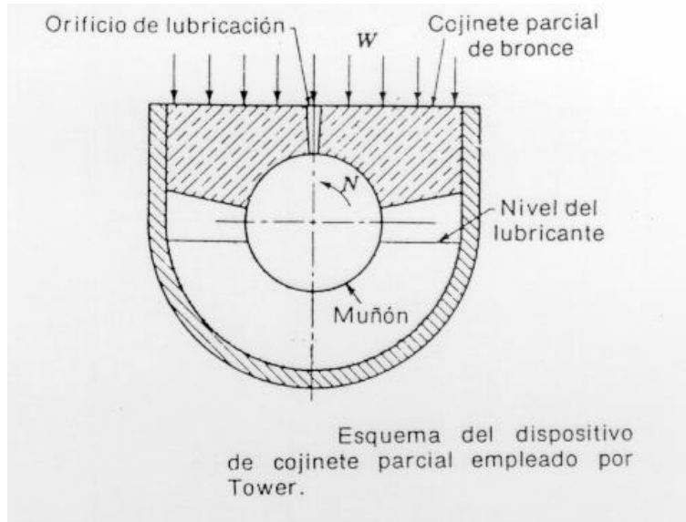
Figura 1.2 Esquema del cojinete de muñón que investigo Tower, obteniendo coeficientes de fricción muy bajos.
