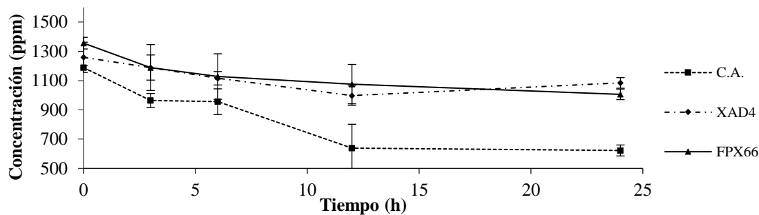
Gráfica 1 Cinética de adsorción para los tres adsorbentes a 25°C, 100 RPM y pH 3.6.
