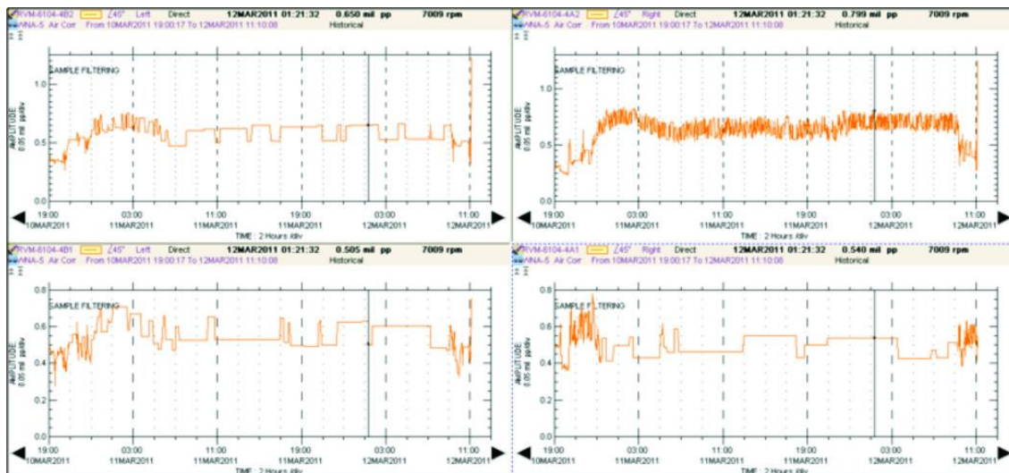
FIGURA 3.7 Las tendencias de la amplitud de la vibración se mantuvieron dentro de los límites aceptables después de implementar los cambios en el diseño del rodamiento.
