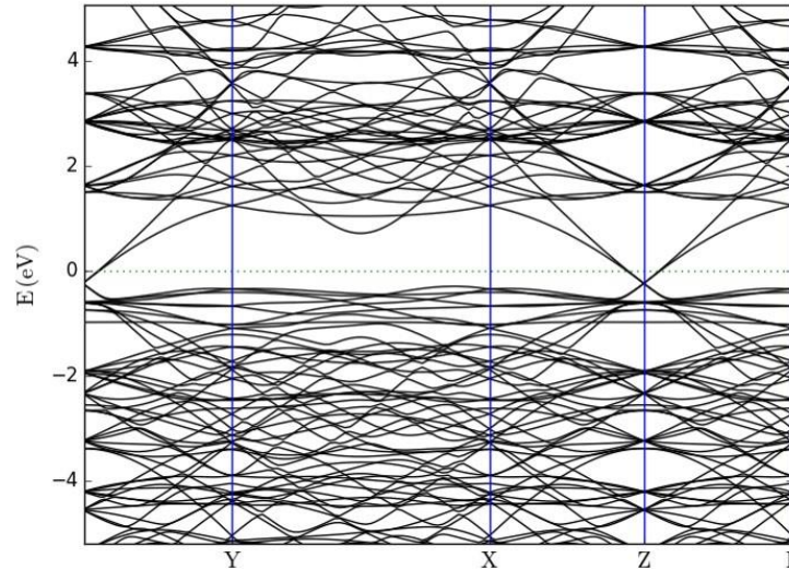
Figura 4. Estructura de bandas de la heteroestructura Gr/WSe 2 .
