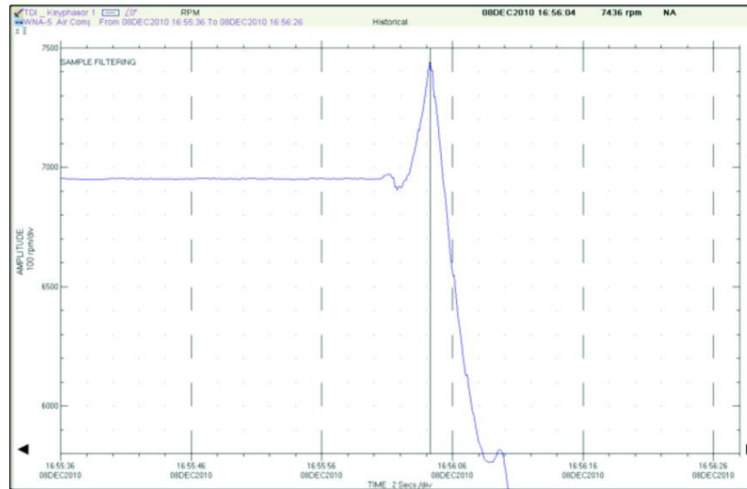
Figura 2.4 La señal de Keyphasor * de la turbina de vapor muestra que la velocidad de la máquina aumentó de 6950 a 7436 rpm antes de caer durante el descenso de la máquina.
