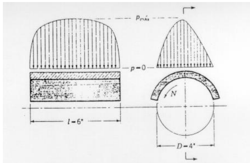
Figura 1.3 Gráficas de distribución de la presión obtenidas por Tower fueron
