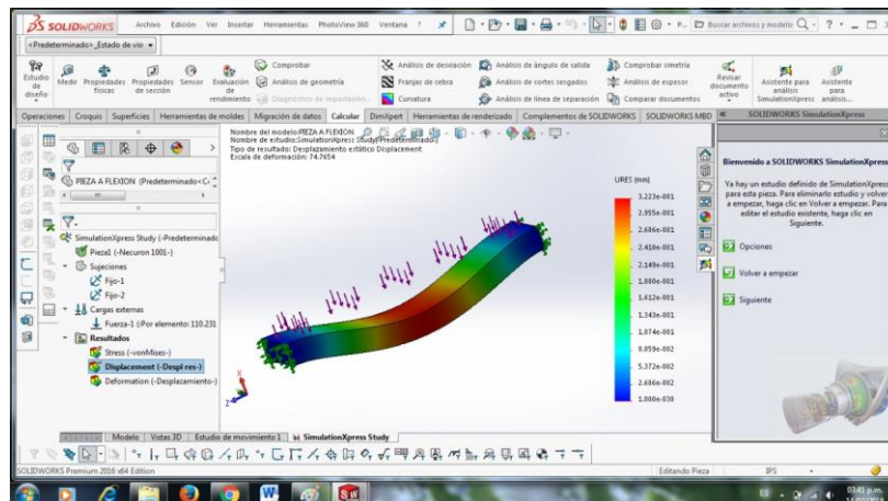
Figura simulación de la probeta de NECURON 1001 de flexión.
