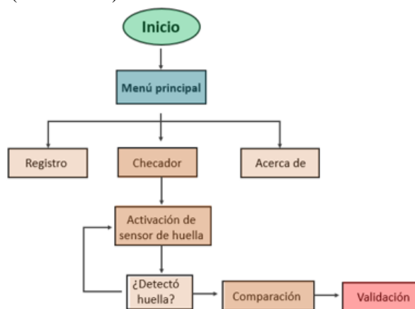
Ilustración 6 Diagrama de Submenú Checador
