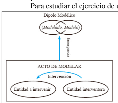
Figura 1. Dipolo modélico (Arrieta y Díaz, 2014)
