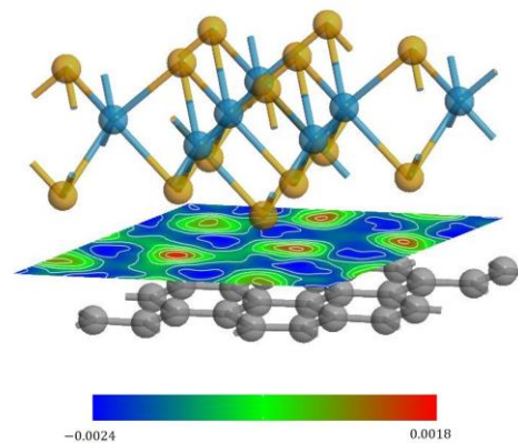
Figura 5. Densidad de carga en la interfaz de la heteroestructura.
