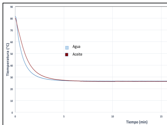
Figura 3. Gráficas de enfriamiento de agua y de aceite
