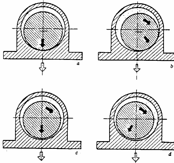
Figura 1 Fases de formación de la película hidrodinámica en un cojinete cilíndrico
