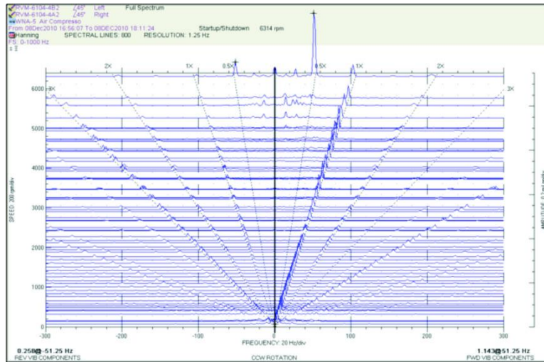
Figura 2.9 El diagrama de cascada de la máquina hacia abajo muestra que los componentes de vibración subsíncrona se disiparon rápidamente a medida que la máquina descendía.
