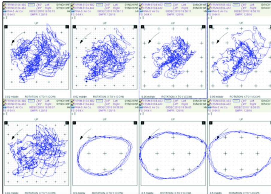
Figura 3.2 Estos diagramas de órbita muestran cómo el movimiento de la línea central del eje cambió de ser muy circular durante la condición de látigo a las 16:56:05 (gráfica inferior derecha), durante un período de movimiento caótico mientras la máquina descendía después del viaje.
