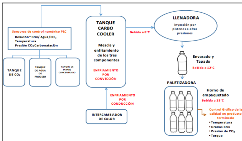
Figura 1. Proceso de envasado de bebidas carbonatadas
