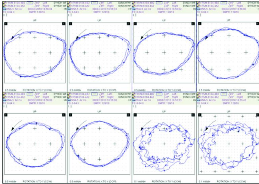
Figura 3.1 Estas gráficas de la órbita muestran los síntomas del azote del aceite que se vuelven más pronunciados desde el movimiento caótico a las 16:55:43 en la esquina inferior derecha, a través de un patrón muy circular que comienza a las 16:56:00 (segundo trazado desde la izquierda en la fila inferior).
