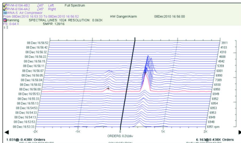
Figura 2.5 frecuencia subsincrónica 0.438X que fue responsable del aumento de las amplitudes de vibración directa.
