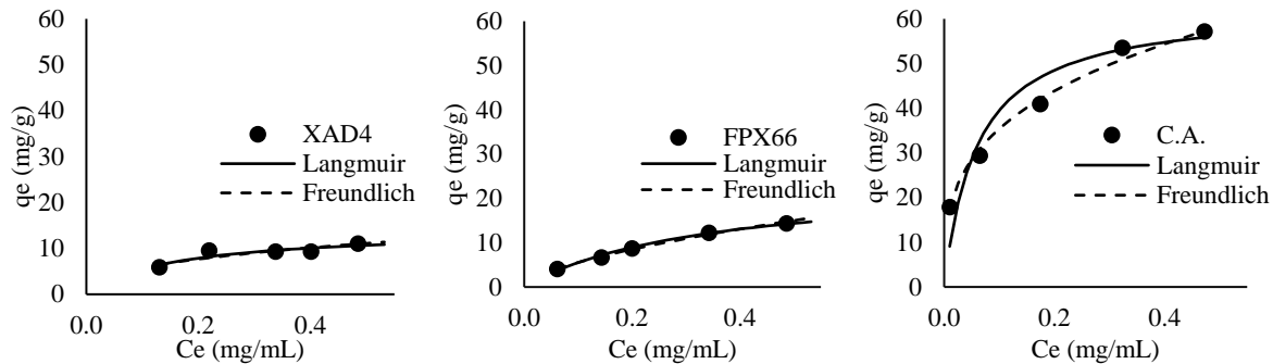
Gráficas 2, 3 y 4 Isotermas a 25°C, pH de 3.6 y 100 RPM para cada adsorbente y ajustes a modelos de Langmuir y Freundlich
