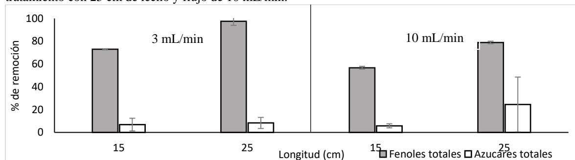
Gráfica 6 Porcentajes de remoción de fenólicos y azúcares totales durante los experimentos de adsorción en columnas de lecho empacado con carbón activado a pH 3.6 y temperatura ambiente.
