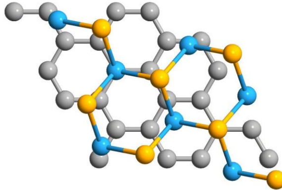
Figura 1. Vista superior de la heteroestructura formada por grafeno y WSe_2 , En gris se muestran los átomos de carbono, en azul los de tungsteno y en naranja los de selenio.
