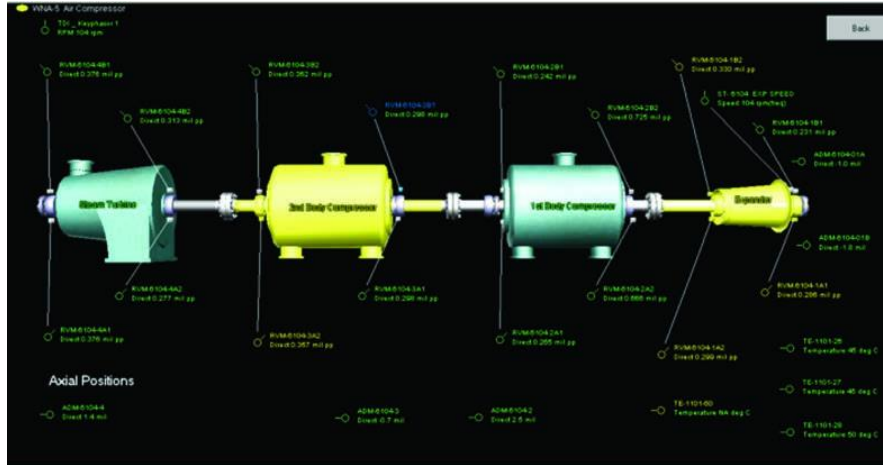
Figura 2 Diagrama de tren de máquina del sistema 1 para el compresor de aire. De izquierda a derecha están la Turbina de vapor, el Compresor del segundo cuerpo, el Compresor del primer cuerpo y el Expansor. Los valores actuales para los parámetros monitoreados se muestran en los bloques de texto.
