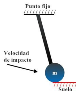
Figura 3. Modelo de péndulo para el análisis dinámico de la rodilla.
