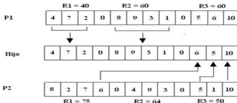
Figura 4. Cruza por intercambio de subsecuencias BRBAX. Fuente: Elaboración propia.
