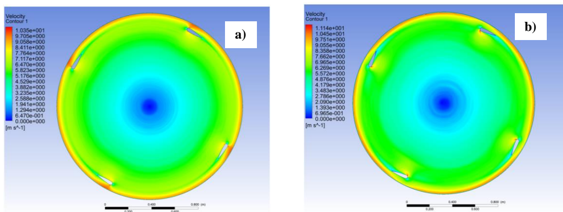
Figura 6 Resultados de los perfiles de velocidad cuando; a) \beta=0 y b) \beta=10
