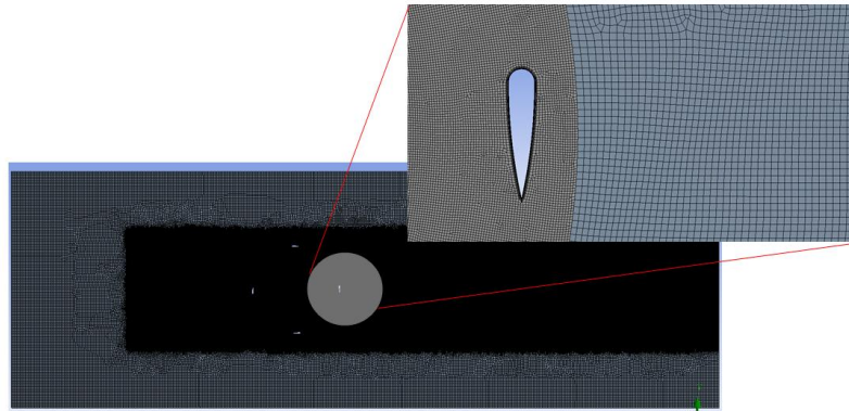
Figura 3. Mallado
