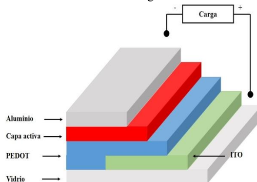
Figura 1 - Esquema de una celda de heterounión orgánica (polímero/fulereno). La capa activa se encuentra entre dos contactos: en la parte inferior se encuentra un electrodo de ITO recubierto con una capa transportadora de huecos PEDOT:PSS y en la parte superior un electrodo de aluminio.
