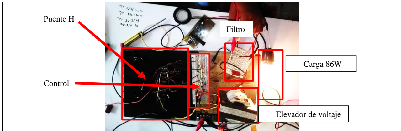
Figura 8 prueba del inversor
