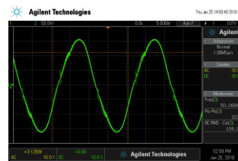
Figura 7 señal senoidal lograda
