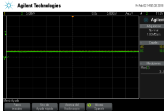
Figura 5 señal de retroalimentación
