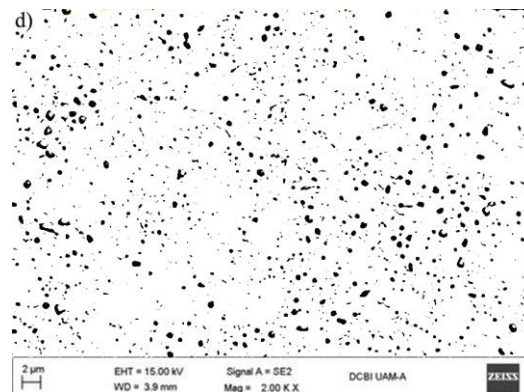
Figura 1d. Micrografía pasador sustituto procesada
