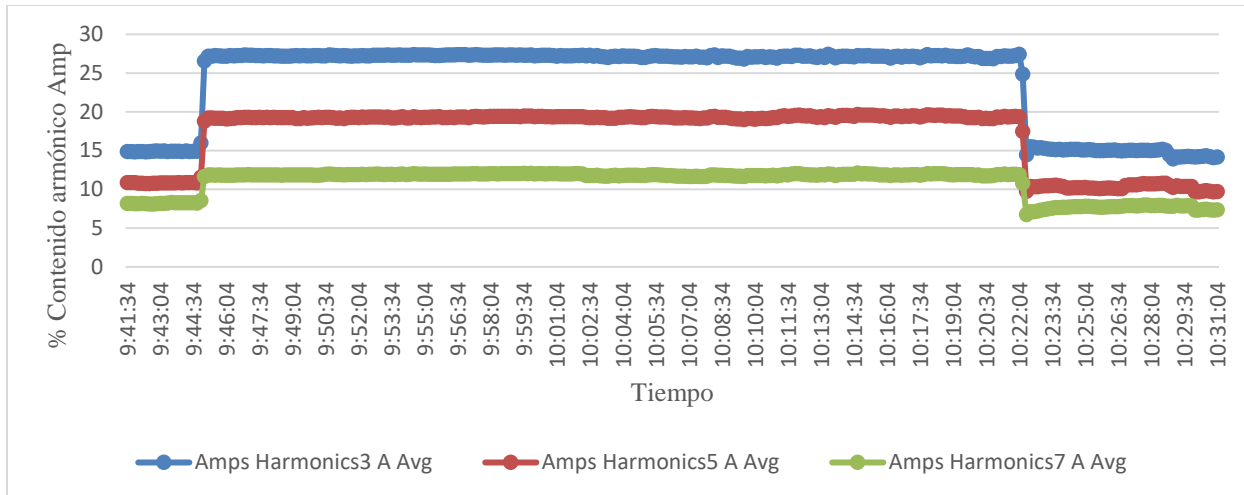
Gráfica 5 – Contenido armónico en la corriente de fase. Valores propios
