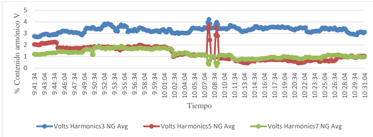
Gráfica 3 – Contenido armónico en el voltaje de neutro a tierra. Valores propios
