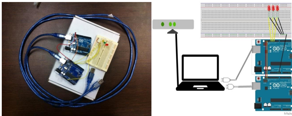
Figura 7. Muestra la forma de la conexión entre los dispositivos
