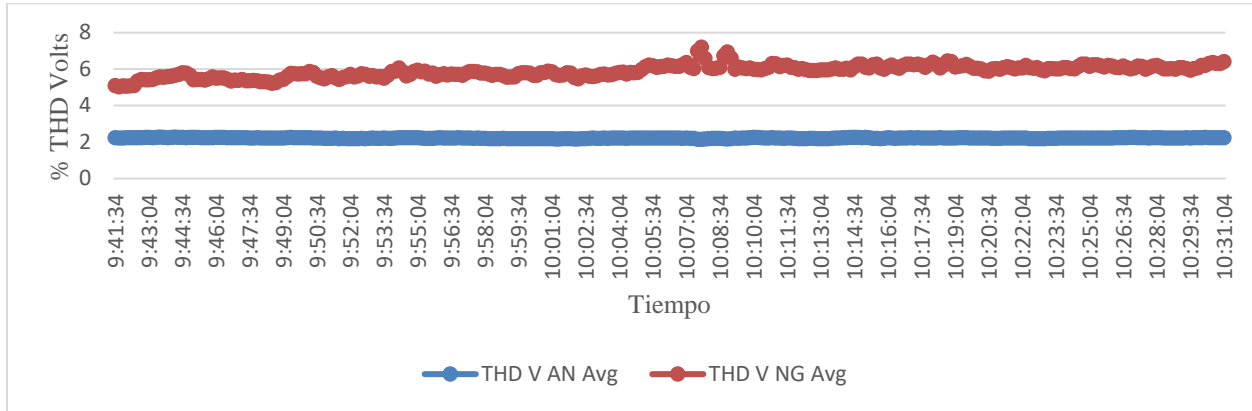
Gráfica 1 - Distorsión Armónica Total (THD) en los voltajes de fase a neutro y de fase a tierra. Valores propios
