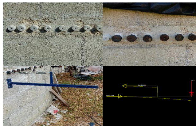
Ilustración 2. Proceso de ensayo de adherencia de muestras de mortero de recubrimiento.
