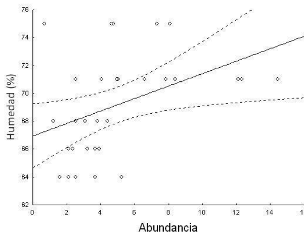
Figura 2. Análisis de regresión entre el porcentaje de Humedad y el total de insectos
