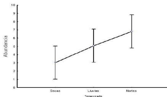
Figura 1. Variación de la abundancia de insectos con respecto a la temporalidad.
