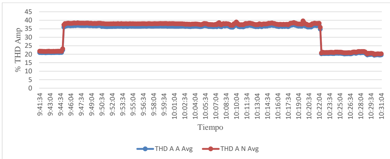
Gráfica 4 - Distorsión Armónica Total (THD) en las corrientes de fase y neutro. Valores propios.
