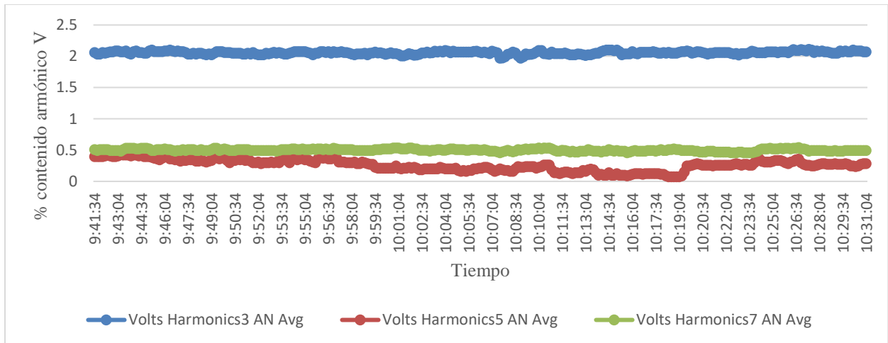
Gráfica 2 – Contenido armónico en el voltaje de fase a neutro. Valores propios.
