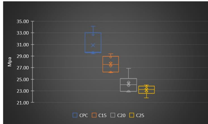
Ilustración 1. Resistencia a compresión de muestras de mortero con sustitución parcial de espuma rígida de poliuretano reciclado.
