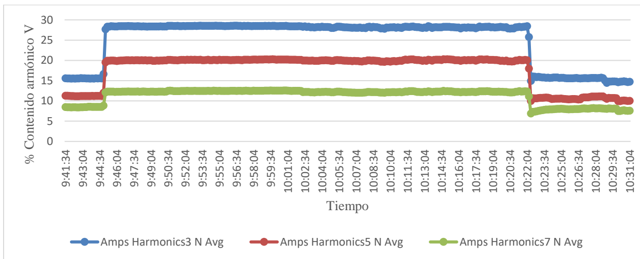
Gráfica 6 - Contenido armónico en la corriente de neutro. Valores propios.
