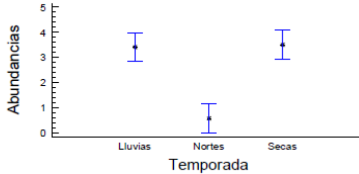
Figura 2. Variación temporal de arañas asociadas a cultivo y selva mediana de acuerdo con el test de Fisher LDS ( p < 0.05 ).
