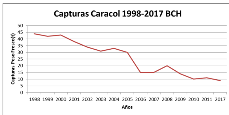
Figura 1. Capturas históricas del caracol rosado en toneladas para Banco Chinchorro (1998-2017)
