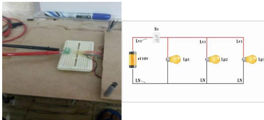
Ilustración 5 Conexión en la protoboard y conexión en paralelo
