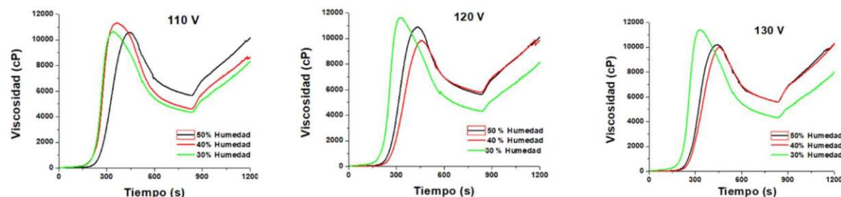
Figura 2. Viscoamilogramas de almidón de papa por calentamiento óhmico a humedades de 30%, 40% y 50% y a voltajes de procesamiento de 110, 120 y 130 volts.
