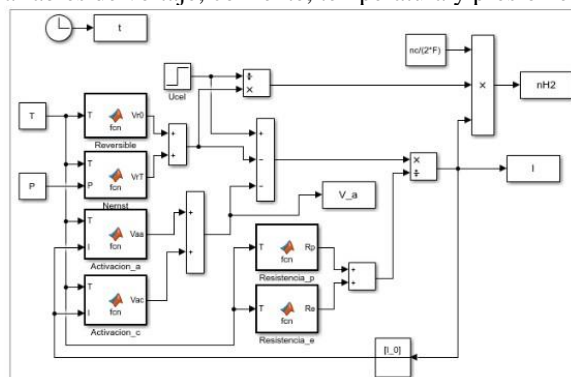
Figura 2. Programación mediante diagrama de bloques
