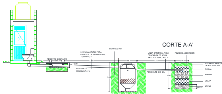
Imagen 2. Planos biodigestor, 2018.
