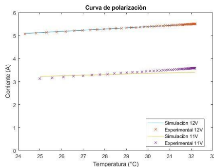
Figura 5. Curva de polarización experimental y simulada a 11V y 12V
