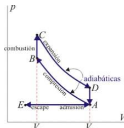
Figura 4. Ciclo Otto de aire normal
