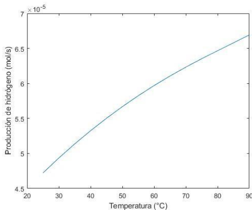
Figura 6. Producción de hidrógeno en función de la temperatura
