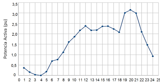
Ilustración 2. Curva de demanda para días hábiles normalizada con base al sistema IEEE 9 nodos Fuente: XM
