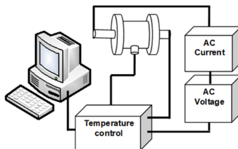
Figura 1 Diagrama esquemático del equipo por calentamiento óhmico utilizado.
