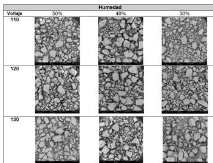
Figura 3. Micrografías de almidón de papa tratados por calentamiento óhmico
