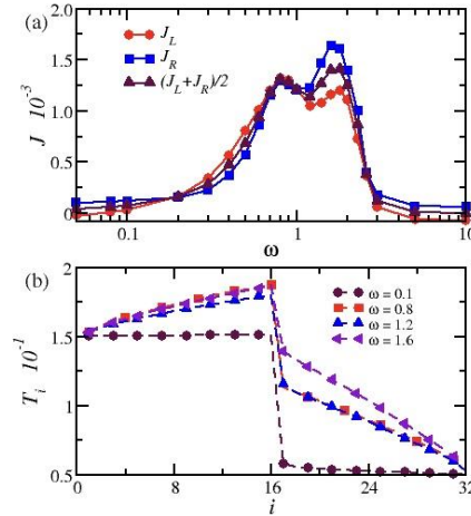
Figura 2. a) Flujo de calor como función de la frecuencia de forzamiento externo. b) Perfiles de temperatura para diferentes frecuencias de forzamiento externo. Los parámetros utilizados son: V_R = 4 , V_L = 5 , k_R = 0.8 , k_L = 1 , \lambda = 0.8 , k_{int} = 0.05 , T_L = 0.15 , T_R = 0.05 , N=32
