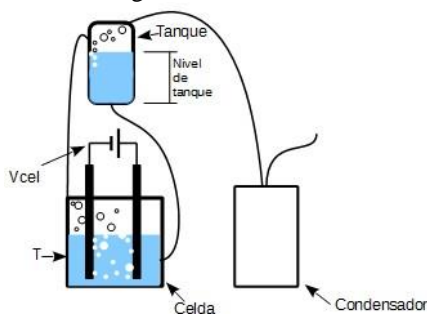
Figura 3 Esquema de instalación experimental
