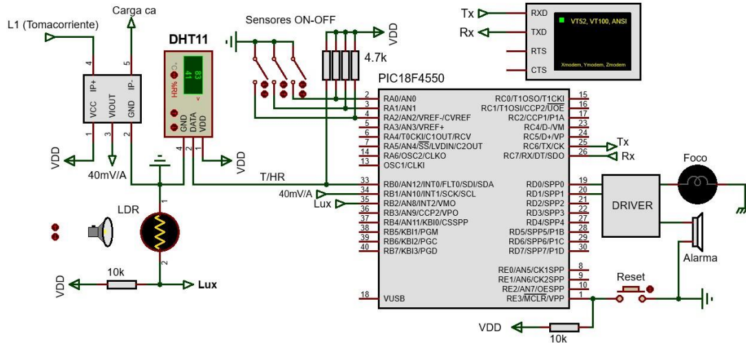
Figura 3. Diagrama esquemático para la medición de parámetros y activación de alarmas.
