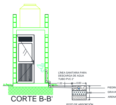
Imagen4. Planos biodigestor, 2018.
