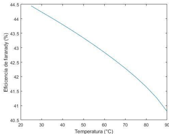
Figura 7. Eficiencia de Faraday en función de la temperatura
