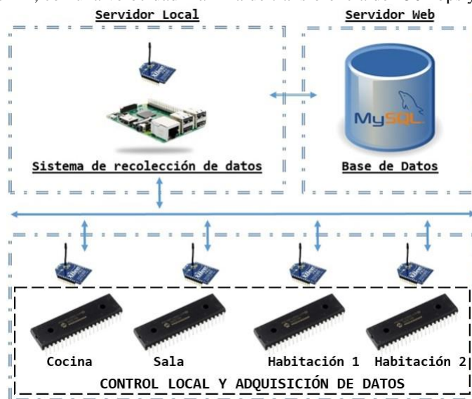
Figura 4. Estructura de la red ZigBee.
