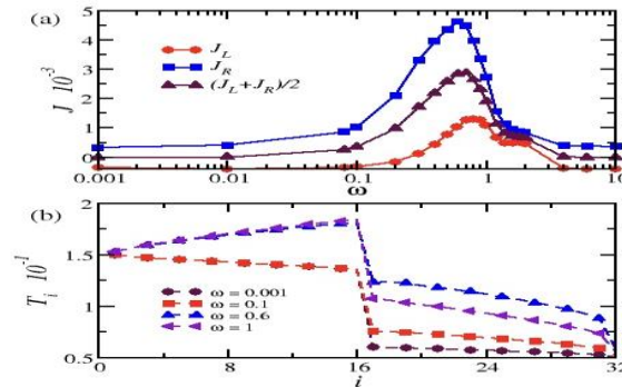
Figura 1. a) Flujo de calor como función de la frecuencia de forzamiento externo. b) Perfiles de temperatura para diferentes frecuencias de forzamiento externo. Los parámetros utilizados son: V_R = 1 , V_L = 5 , k_R = 0.2 , k_L = 1 , \lambda = 0.2 , k_{int} = 0.05 , T_L = 0.15 , T_R = 0.05 , N=32
