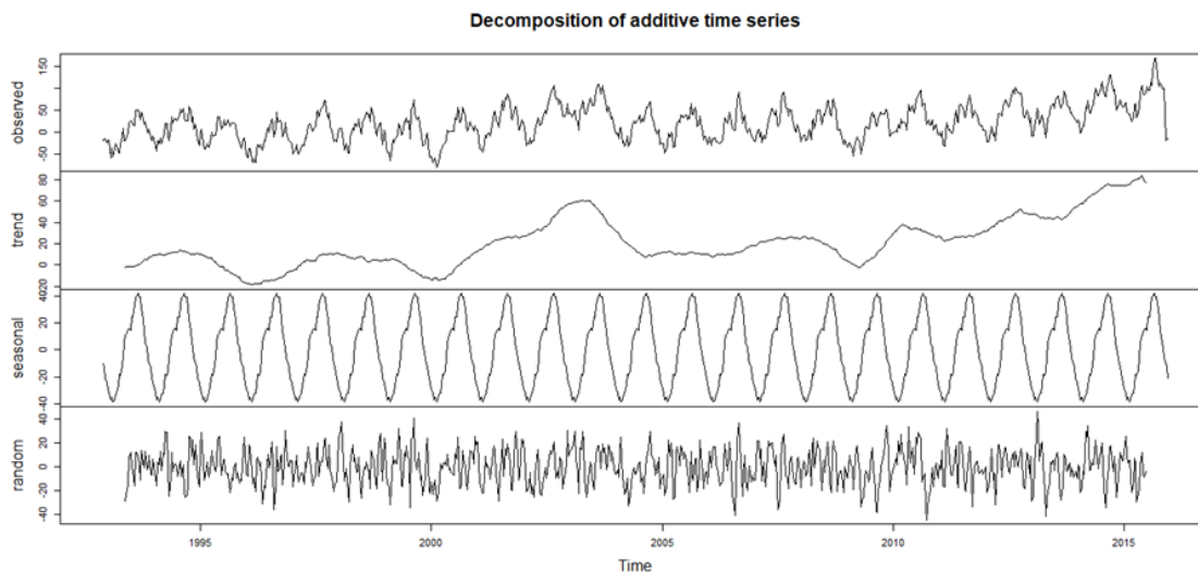
Figura 1. Componentes de la serie de tiempo aplicando Fourier para el periodo 1993-2015 de la región del Mar Caribe.
