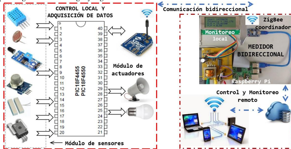
Figura 5. Diagrama del sistema propuesto para la gestión energética y seguridad doméstica.
