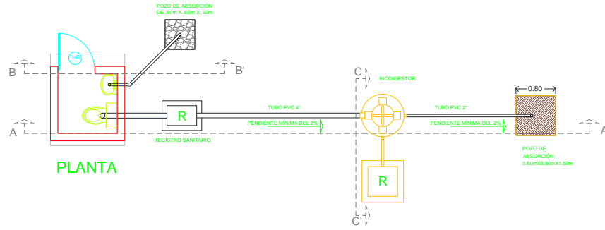
Imagen 1. Planos biodigestor, 2018.
