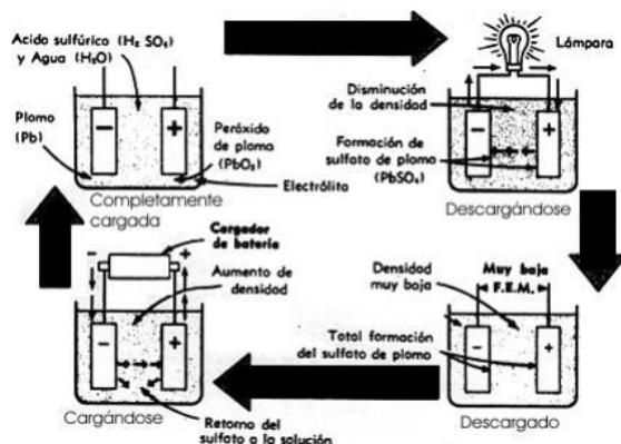
Ilustración 3 Funcionamiento de batería plomo ácido
