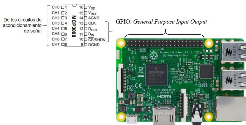
Figura 2. Conexión del convertidor ADC con las entradas GPIO del módulo Raspberry Pi.
