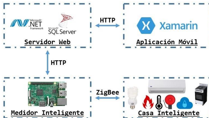
Figura 1. Diagrama a bloques del sistema para la gestión energética y seguridad doméstica.
