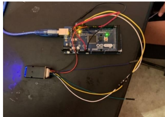
Figura 7. Conexión del lector y la placa.
