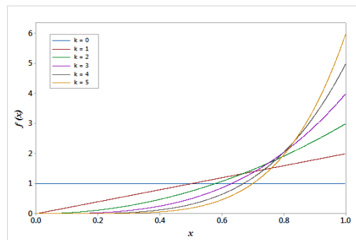
Figura 1. f_{X^k}(x) , para k = 0,1,2,3,4,5 .
