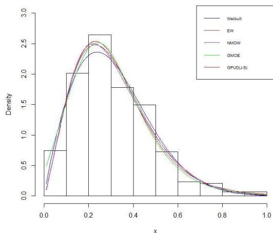
Figura 3. Ajuste de la FDP para W, EW, NMOW, GMOE y DUPG_{(J-S)} para datos Covid-19.
