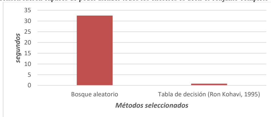
Figura 5. Tiempo de construcción de modelo para 500 choferes ~ 32 mil registros.
