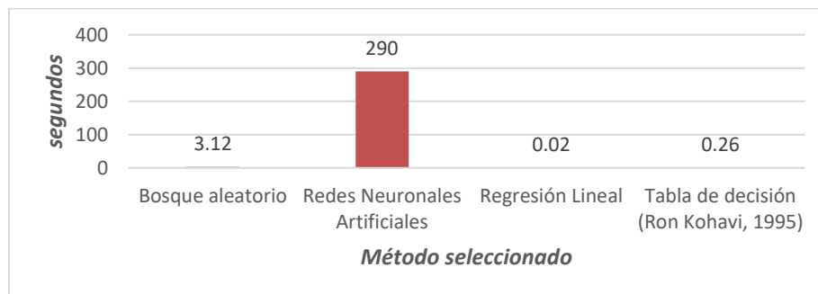
Figura 2. Tiempo de construcción de modelo para 50 choferes ~ 9 mil registros.
