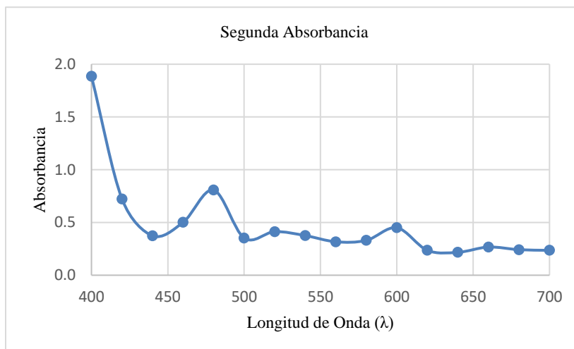
Figura 2. Curva de calibración en las siguientes condiciones: Secado Luz Solar, curado con Alcohol Isopropílico, segunda Absorbancia. Sumergido Fosfato, absorbancia de 0.217 a \lambda igual a 640nm
