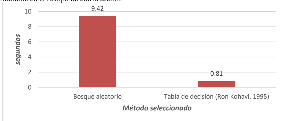
Figura 4. Tiempo de construcción de modelo para 200 choferes ~ 21 mil registros.
