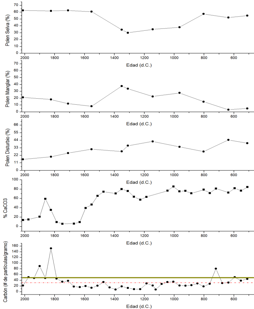
Figura 2. Comparación de las sumas de polen de vegetación de selva, manglar y disturbio, y la curva de carbonatos de calcio (CaCO 3 ) (Rosas, 2018), con el número de partículas de carbón expresado en partículas por gramo. La línea punteada representa el promedio de los últimos 1500 años (33 p/g). La línea verde marca el valor mínimo de carbón (p/g) empleado para identificar eventos de incendios.
