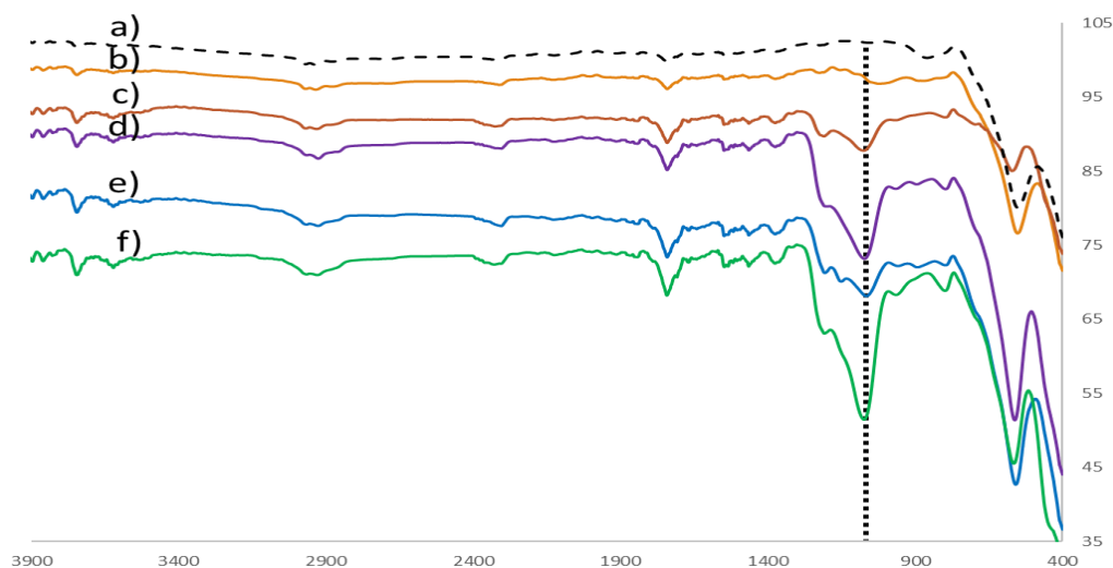
Figura 2. Espectros infrarrojos de los sólidos: a) \text{Fe}_3\text{O}_4 y \text{Fe}_3\text{O}_4\text{-SiO} a b)4, c)6, d)8, e)16 y f)24 h.
