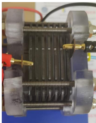
Figura 1. Celda de combustible con escalamiento a 7 ensambles membrana/electrodos.
