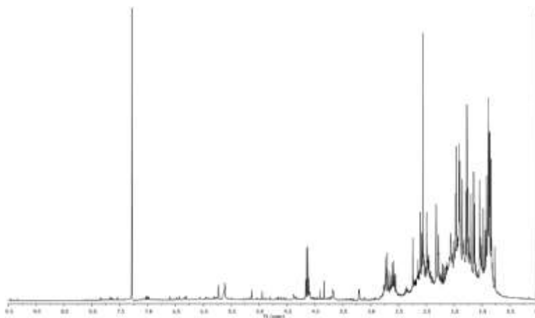
Figura 6. Espectro de RMN de ^1\text{H} del extracto etanólico F2 [AcOEH] (400 MHz, \text{CDCl}_3 )
