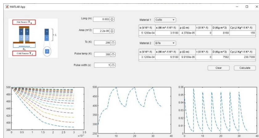
Figura 5. Gráficas del entorno digital para una L = 3 \text{ mm} .
