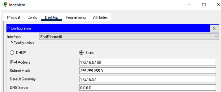
Figura 5. Simulación de configuración de dirección IP.
