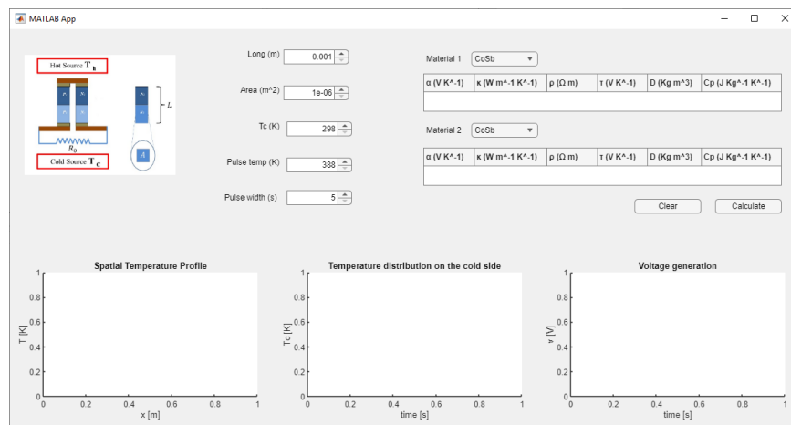
Figura 3. Entorno digital (aplicación) para el analisis de termoelementos.
