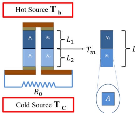
Figura 1. Modelo de generador termoelectrico segmentado (STEG)
