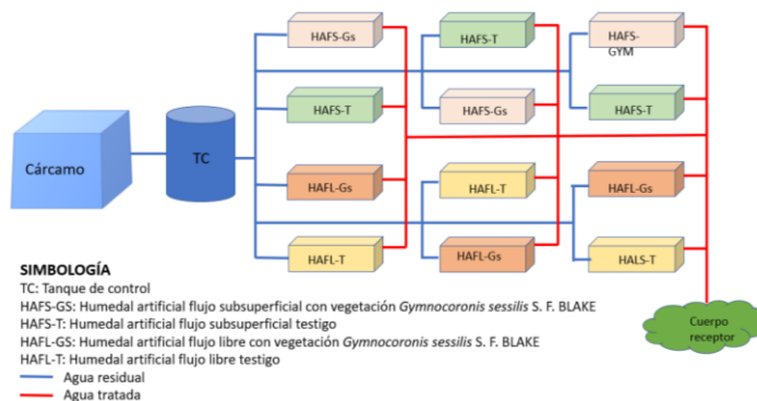
Figura 2. Esquema de distribución de los humedales artificiales. Comentarios Finales
