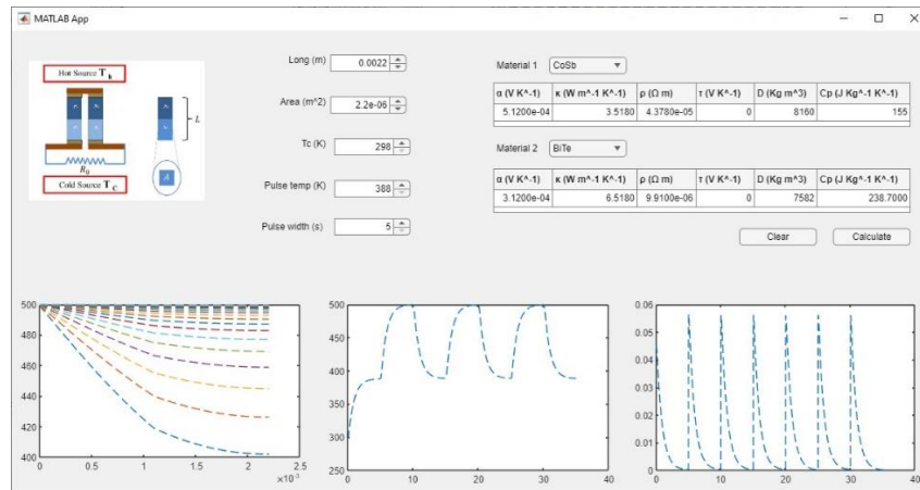
Figura 4. Validación de resultados mediante el entorno digital.
