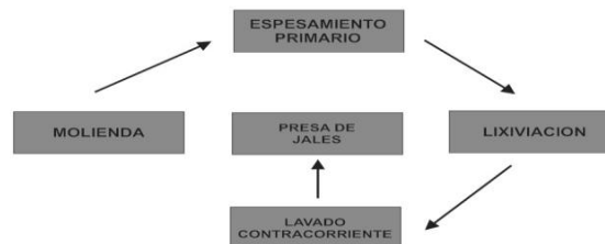
Figura 2. Flujo del proceso de lixiviación de la mina “la parrilla”, Durango.
