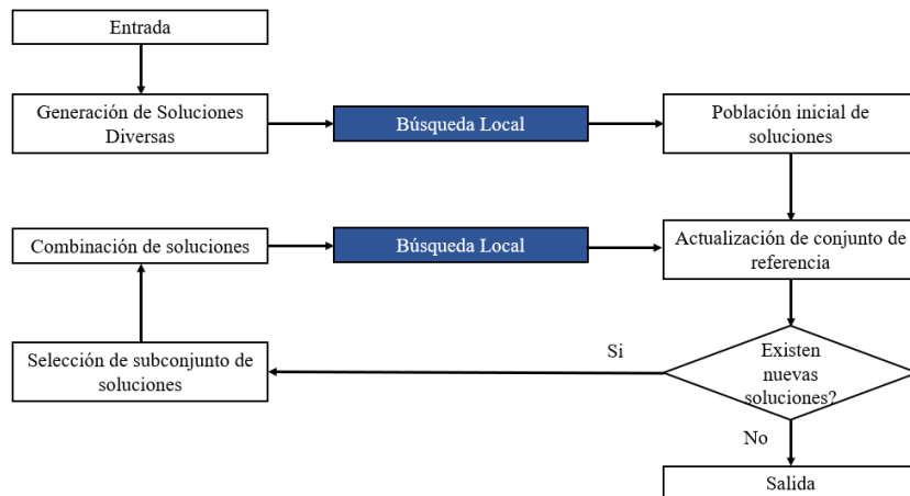
Figura 5. Diseño del algoritmo Scatter Search
