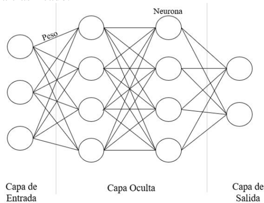
Figura 1. Estructura de un ANN
