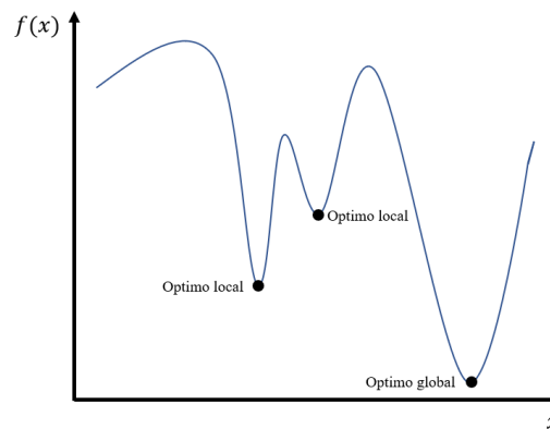
Figura 3. Estancamiento del descenso de gradiente
