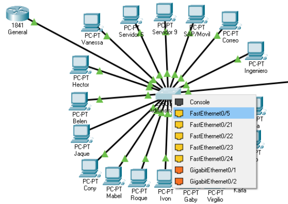
Figura 4. Configuración de puertos del switch
