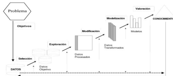
Figura 1: Proceso SEMMA
