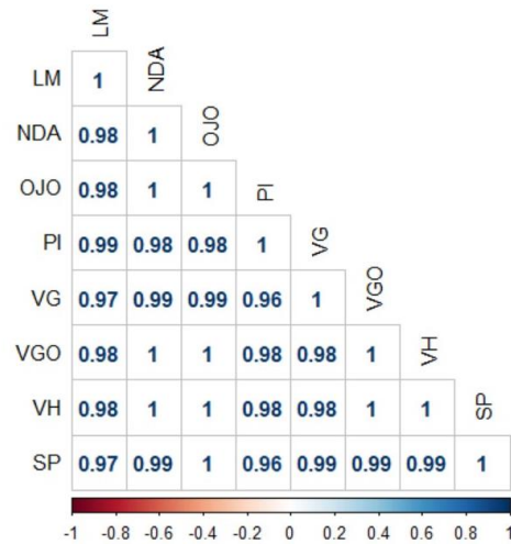
Fig. 3. Colinealidad de las variables del modelo.
