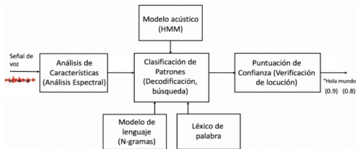
Figura 2. Diagramas de bloques de un sistema global de reconocimiento de voz.
