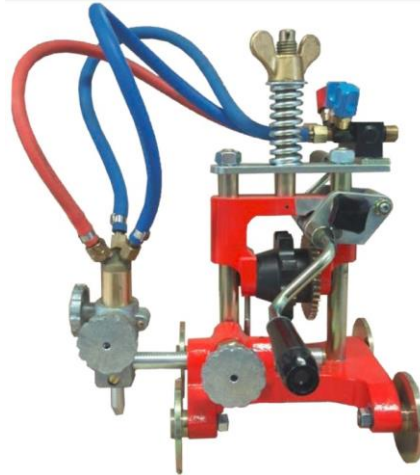
Figura 6 Máquina de corte de tubería Oxicorte
