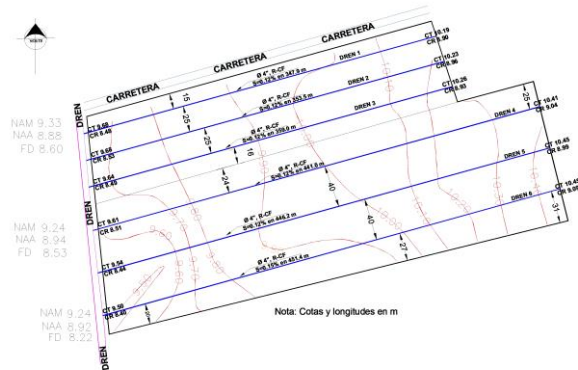
b) Sistema de drenaje agrícola subterráneo
