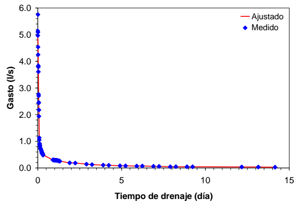
Figura 2. Evolución del gasto de agua total evacuado del suelo por la línea de drenaje central asociada a la separación entre drenes de 25 m ( \ell = 353.2.20 \text{ m} y P_d = 1.20 \text{ m} ).
