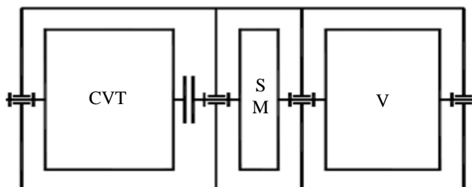
Figura 1. Sistema de regeneración M-KERS de la empresa automotriz Volvo
