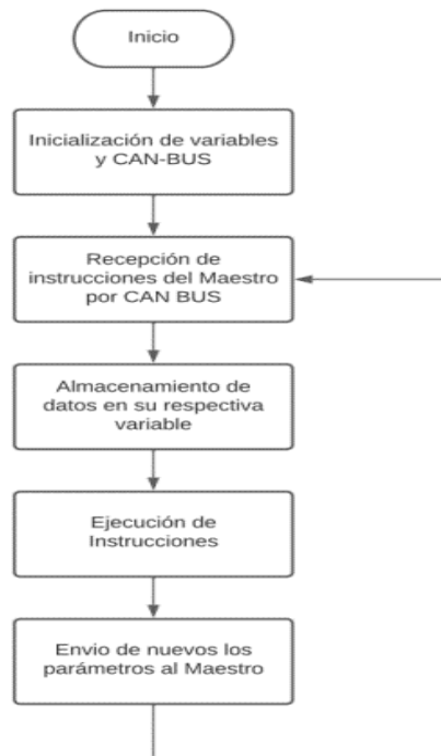
Figura 2. Diagrama de flujo del nodo 1.
