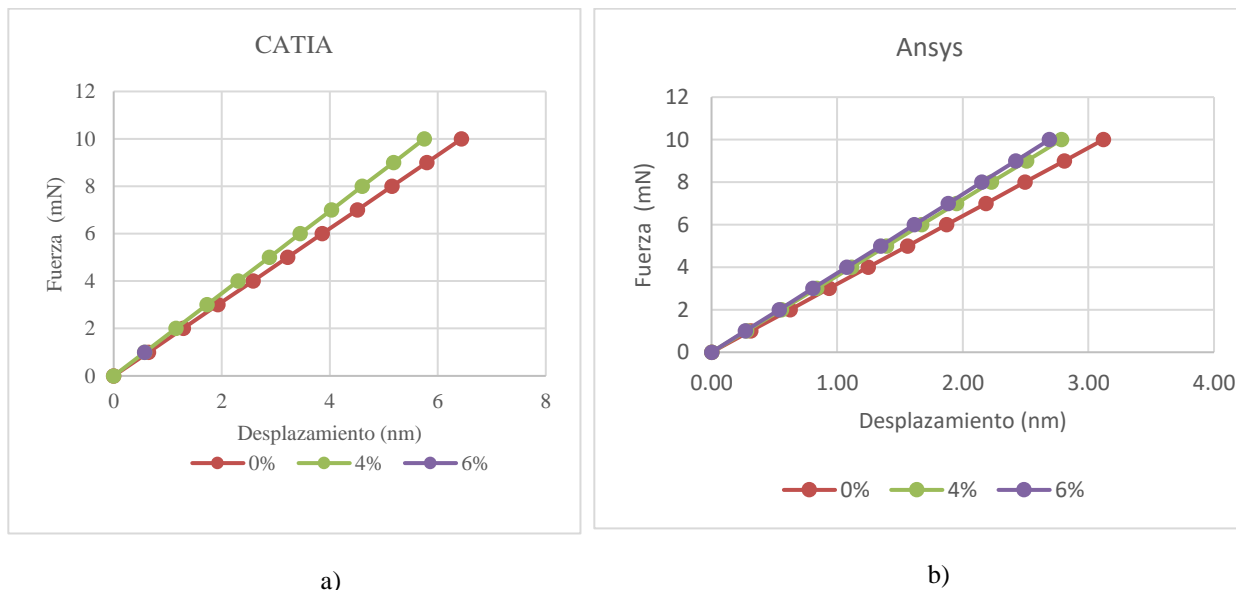
Figura 6. Gráfica de Carga-Desplazamiento a) Catia, b) Ansys
