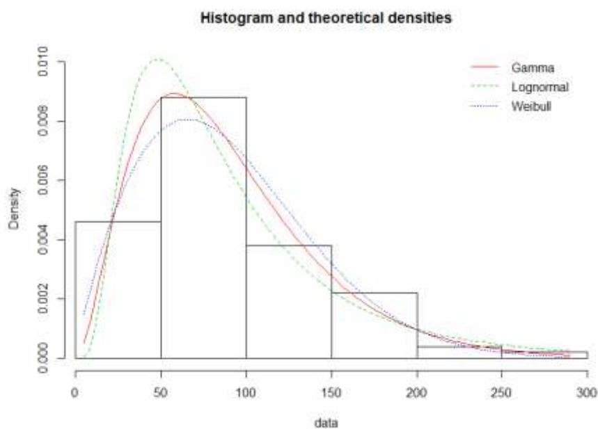
Figura 1 Histograma de los Datos y las Densidades Teóricas
