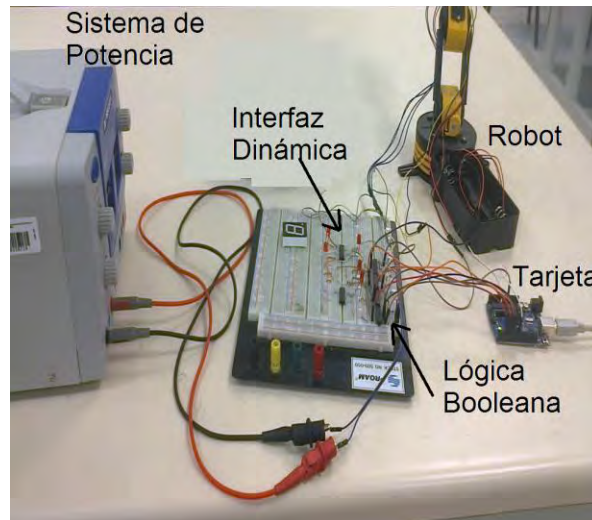
Figura 7. Modelo real
