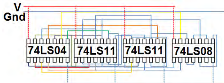
Figura 5. Diagrama Lógico
