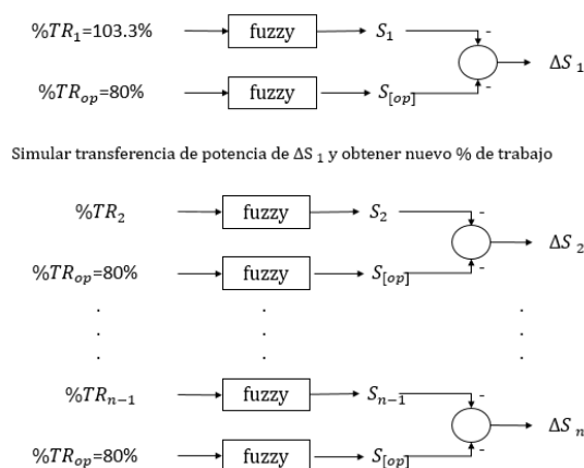
Figura 4.- Algoritmo para inferencia de potencia óptima a transferir por lógica difusa.
