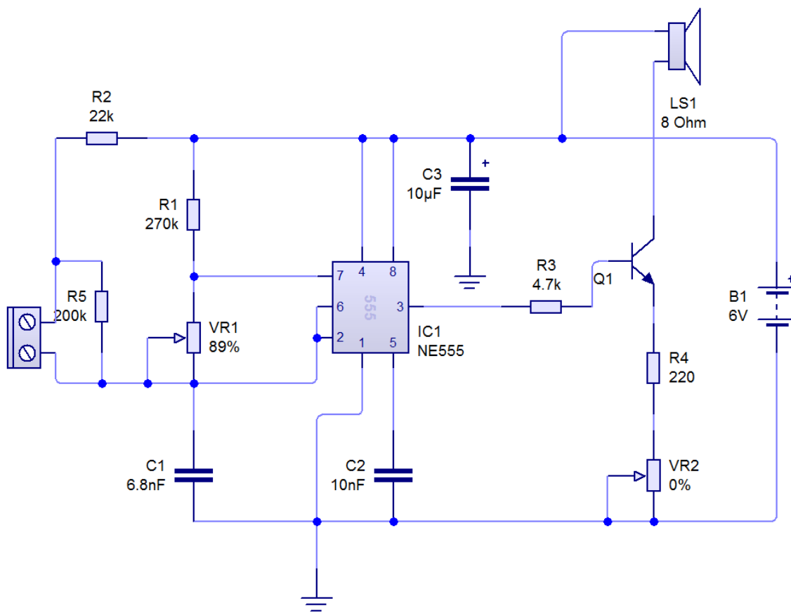
Figura 3. Diagrama esquemático del “estresímetro”.
