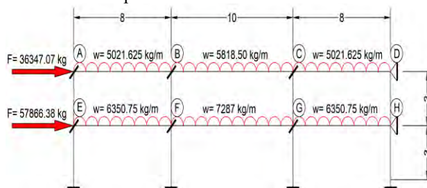
Figura 2. Planteamiento de un marco con continuidad geométrica. Por autores.
