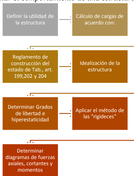
Figura 1. Pasos para determinar el comportamiento de una estructura. Por autores.
