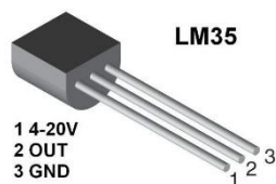
Fig. 3.Sensor de Temperatura LM35
