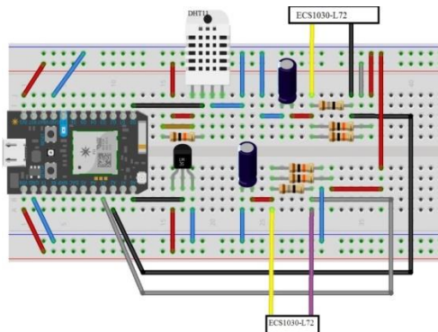
Figura No. 4. Circuito montado en Protoboard realizado en Fritzing.
