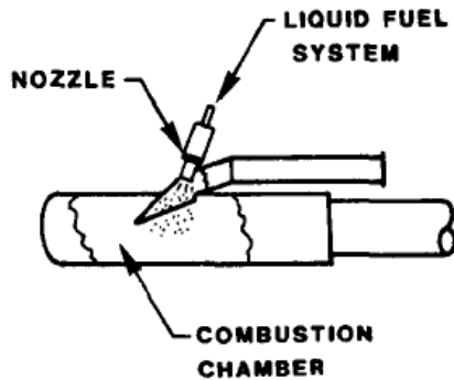
Figura 10. Persechino pulsorreactor 1957. Imagen tomada de (Putnam et al., 1986).
