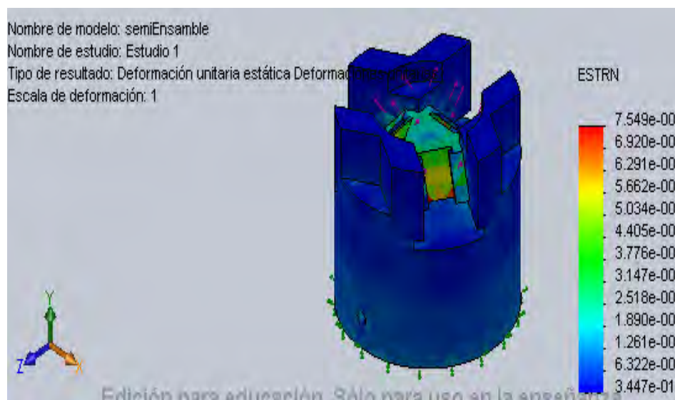
Figura 7 análisis de deformación unitaria estática sobre la base del gripper
