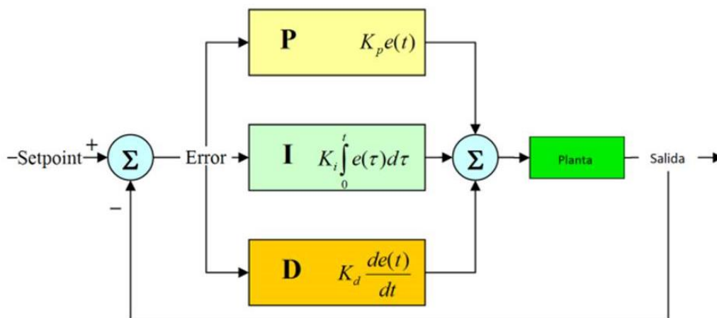
Figura No. 1. Diagrama de Retroalimentación PID
