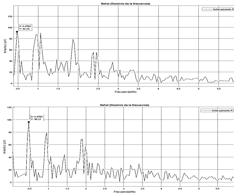
Figura 5: Espectro de frecuencia aplicada al parpadeo dentro de un rango de 0 a 6 Hz, muestras de frecuencias dominantes.
