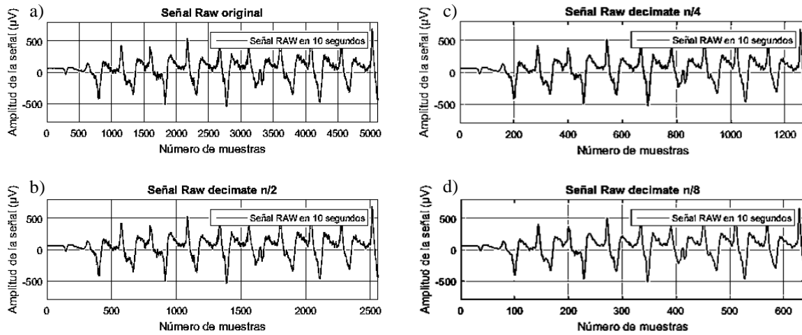
Figura 3: Patrón obtenido realizando un parpadeo, a) Señal Raw original, b) Diezmado con factor de 2, c) Diezmado con factor de 4 y d) Diezmado con factor de 8.
