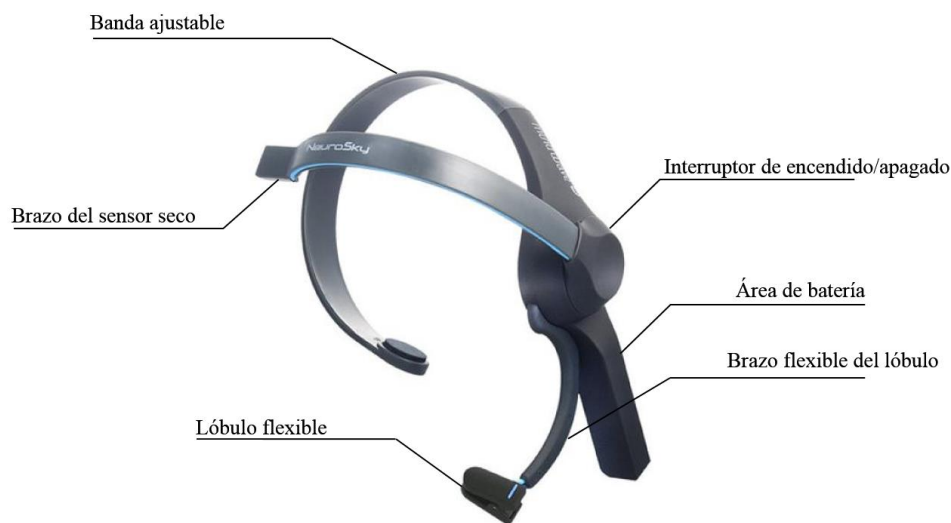
Figura 1: Diseño y partes principales del MindWave Neurosky MW003.
