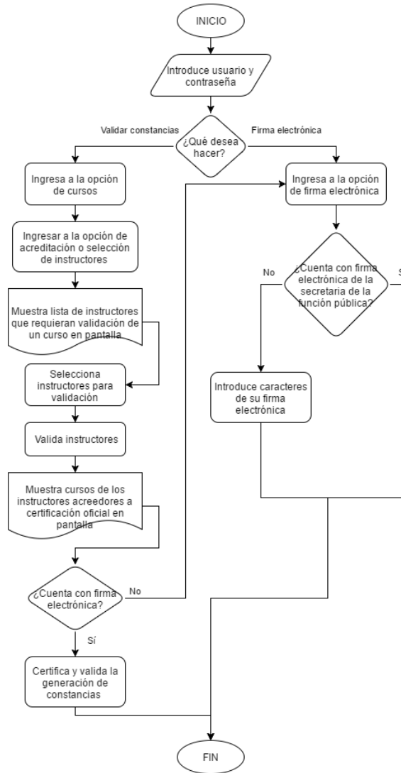
Figura 5 - Diagrama de flujo de funciones del Presidente
