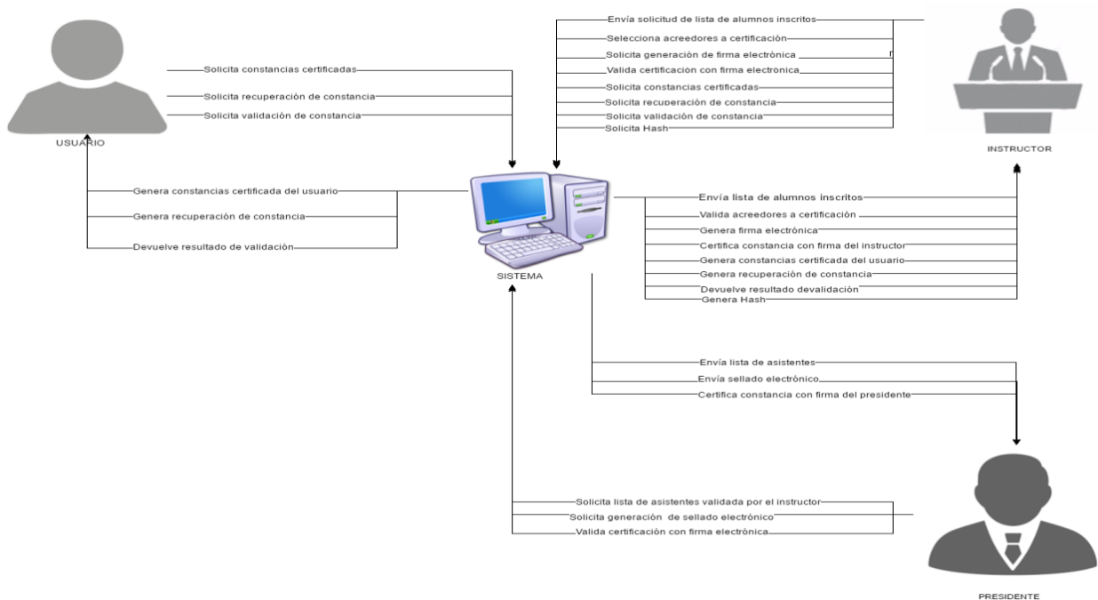
Figura 2.-diagrama de Contexto del Sistema
