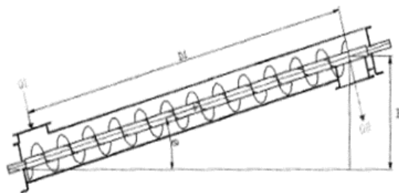
Ilustración 4 Tornillo sin fin inclinado
