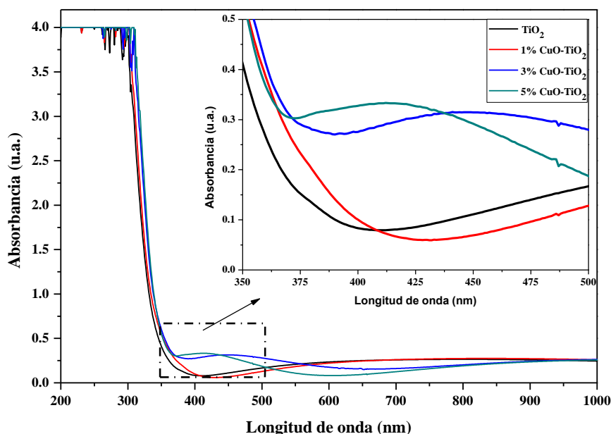
Figura 3.- Espectros de absorbancia UV-vis de las películas delgadas de TiO 2 en diferentes concentraciones de CuO.
