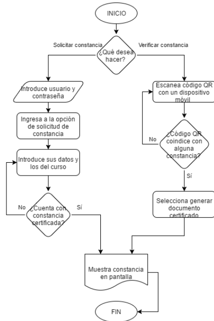
Figura 3 - Diagrama de flujo de funciones del usuario
