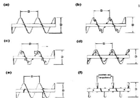
Ilustración 8 sin fin por su forma
