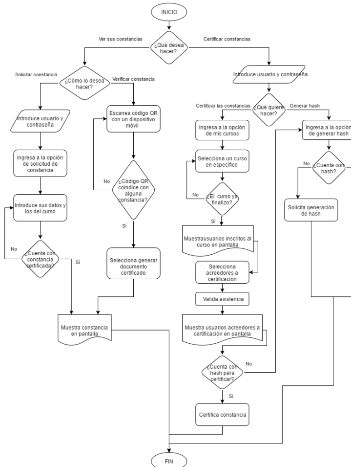
Figura 4 - Diagrama de flujo de funciones del Instructor
