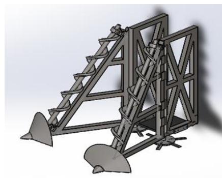
Ilustración 18.- Diseño del implemento
