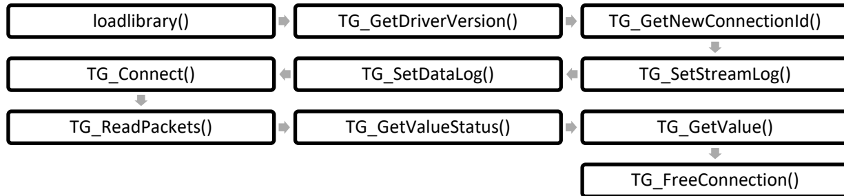
Figura 2: Protocolo general para la conexión de Neurosky Mindwave MW003 con MATLAB.
