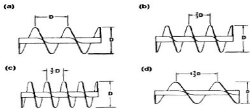
Ilustración 7 tipos de sin fin por su paso
