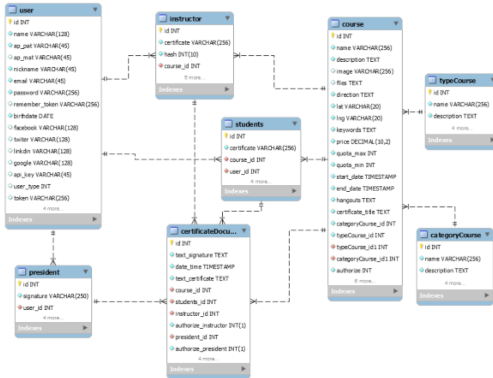
Figura 7 – Diseño de la base de datos
