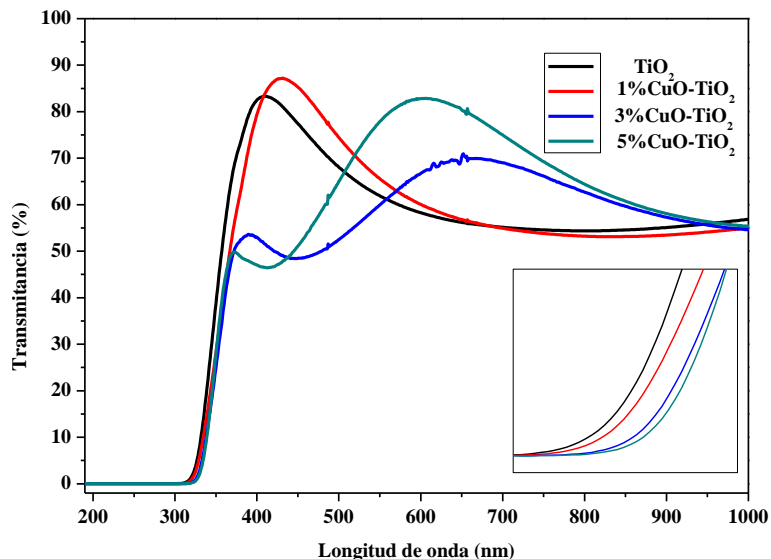
Figura 2.- Espectros de Transmitancia UV-vis de las películas delgadas de TiO 2 con variación del %CuO.
