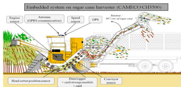
Ilustración 1 Máquina cosechadora de caña de azúcar.
