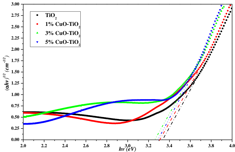
Figura 4.-Grafica de (\alpha h\nu)^{1/2} vs h\nu de transición indirecta de películas de \text{TiO}_2 y 1,3 y 5% \text{CuO-TiO}_2 .
