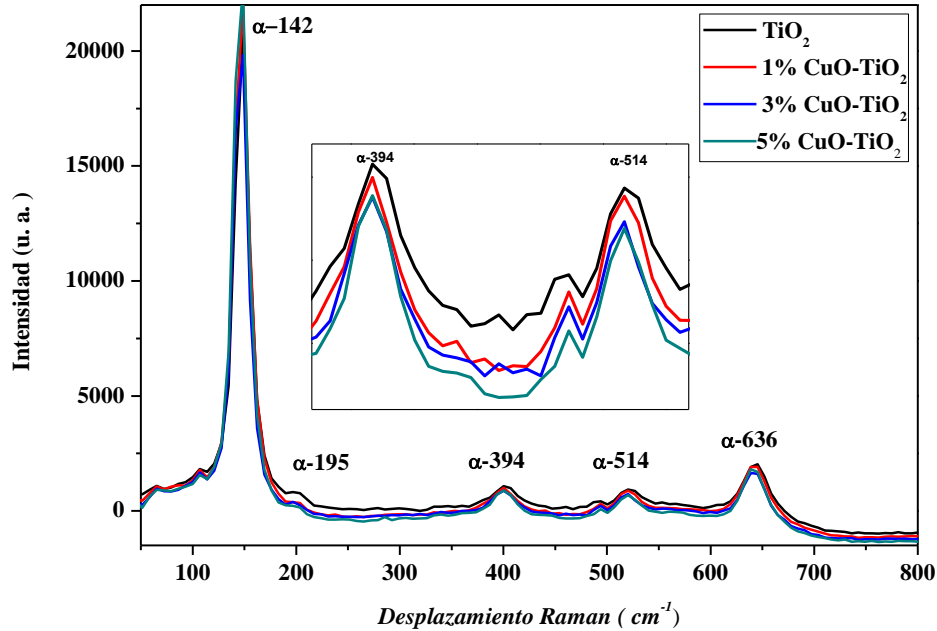
Figura 1.-Respuesta Raman de las diferentes películas %CuO-TiO 2
