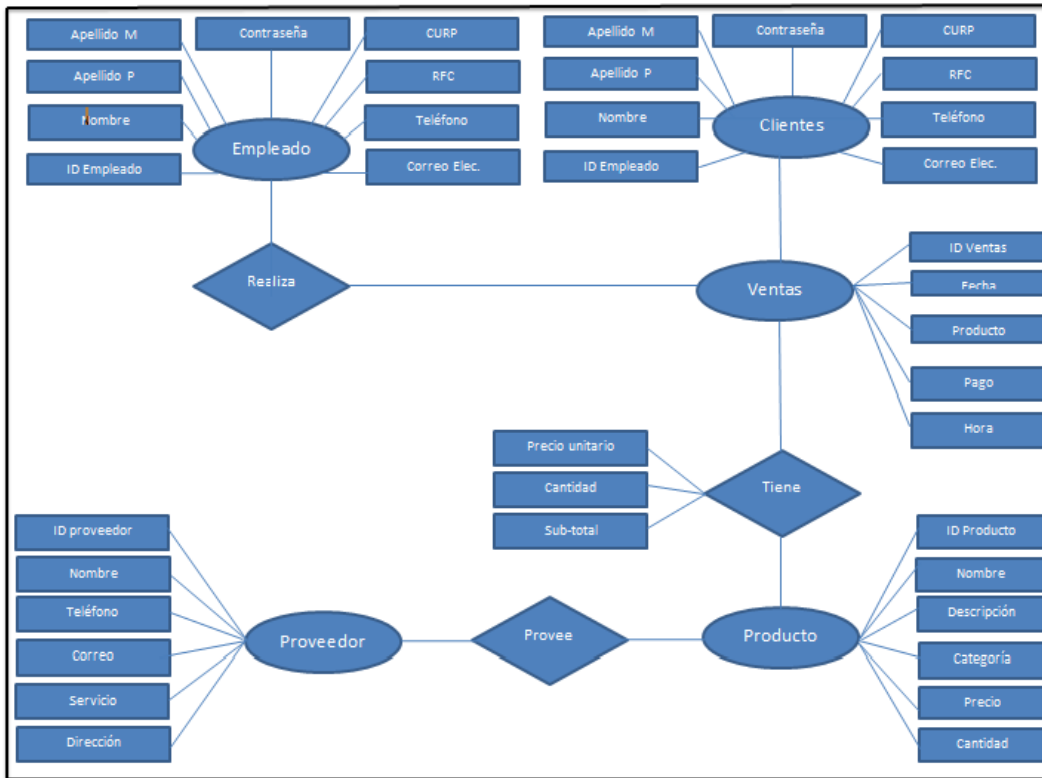
Trasformación modelo Entidad-Relación a código Fuente: Sanchez A. & Rodriguez J. (2016)
