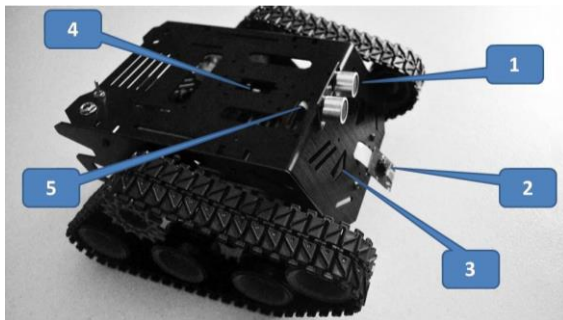
Figura No. 8. Estructura Física del Robot.
