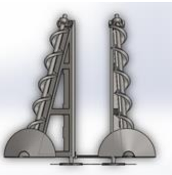
Ilustración 19.- Vista Frontal
