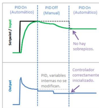
Figura No. 11. Transición de Manual a Automático.
