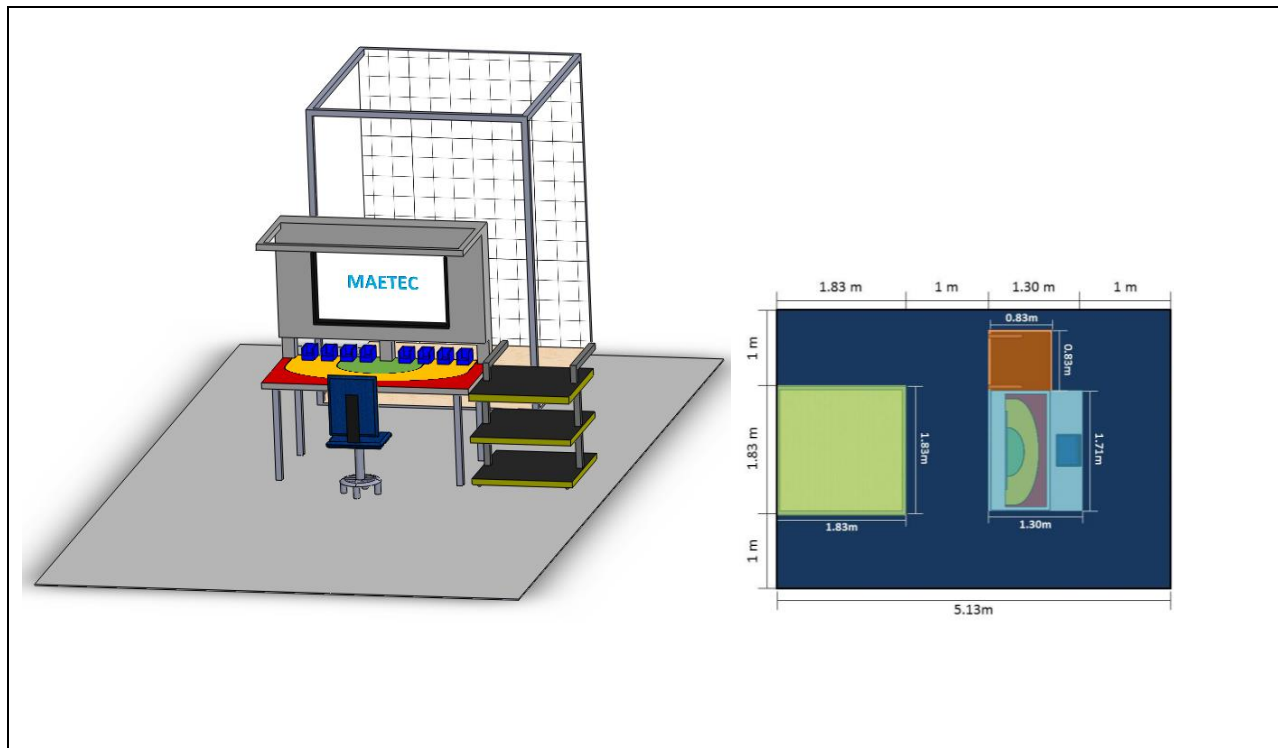
Figura 4. Diseño estructural del módulo (Hardware) y sus dimensiones.
