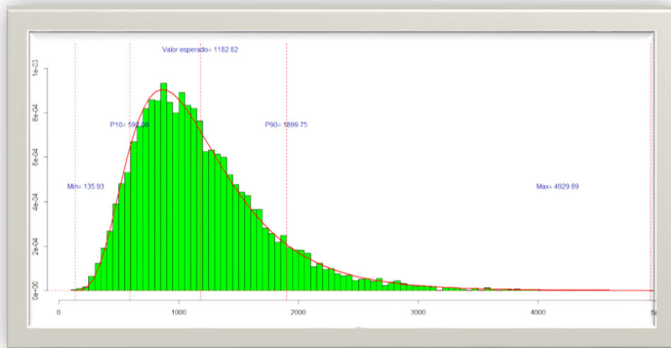
Imagen No. 5 Resultado final de la estimación de la tasa inicial de producción Qoi.
