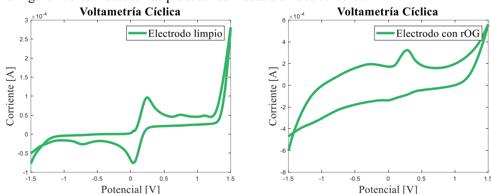
Figura 1. 5 a) voltametría cíclica del sensor limpio y b) del sensor con rOG
