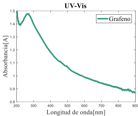
Figura 1. 3 Espectroscopia UV-Vis realizada al producto obtenido
