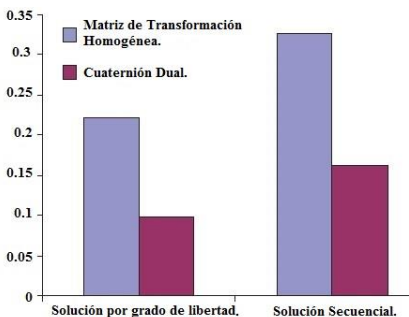
Fig. 7. Gasto computacional entre cada método cinemático.
