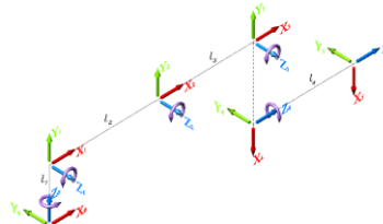
Fig. 2. Sistemas coordenados en cada articulación.
