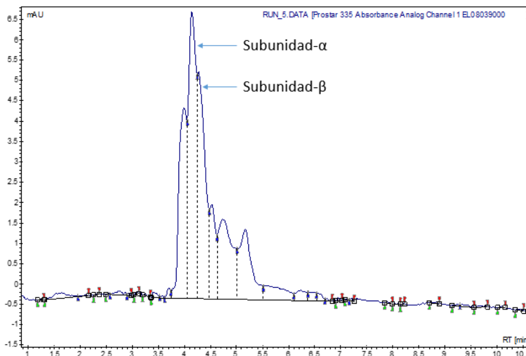
Figura 3. Cromatograma del extracto de ficobiliproteínas. Se observan 2 picos característicos correspondientes a las subunidades de la C-PC.
