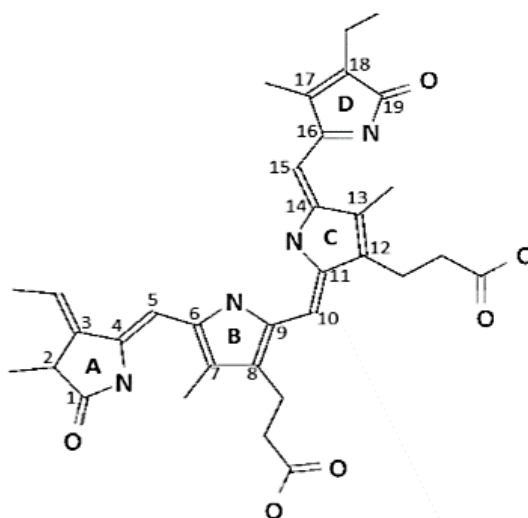
Figura 2. Estructura de la ficocianobilina, el grupo prostético de las ficobiliproteínas C-PC y APC. El sistema tetrapirrólico está conformado por cuatro anillos (A, B, C y D) que dan lugar a un compuesto con insaturaciones conjugadas (Tomado de Llopiz et al. , 2016).
