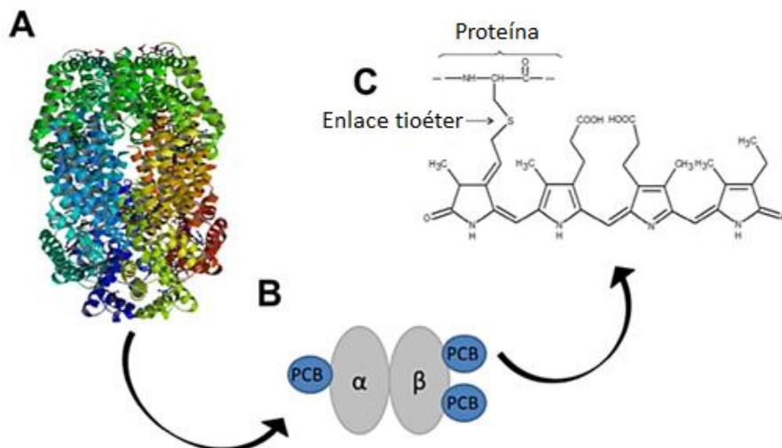
Figura 1. Estructura de la C-PC. (A) Estructura cristalina de la C-PC de la cianobacteria Spirulina platensis en su forma de hexámero. (B) Representación esquemática del ensamblaje de la C-PC, la cual está compuesta por dos subunidades proteínicas (cadenas \alpha y \beta ). Una molécula de ficocianobilina está enlazada a la subunidad \alpha y 2 moléculas de ficocianobilina están enlazadas a la subunidad \beta . (C) Estructura química de la ficocianobilina, grupo cromógeno de la C-PC. Imagen tomada de PDB ID 1GHo (2011).
