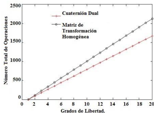
Fig. 6. Comparación entre las técnicas para determinar cinemática.
