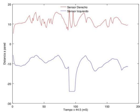
Figura 7. Control Proporcional Difuso; datos de distancia de los sensores izquierdo y derecho durante el desplazamiento
