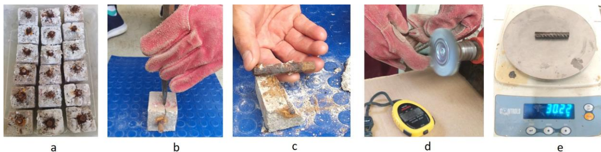
Figura 3. Procedimiento para calcular de la pérdida de masa, a) probetas agrietadas, b) extracción de varillas, c) varilla corroída, d) limpieza y e) registro de masa
