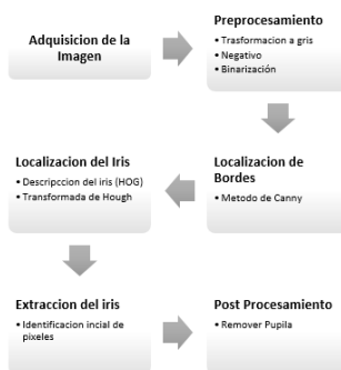
Figura 1. Fases para la segmentación del iris, utilizando la transformada de Hough
