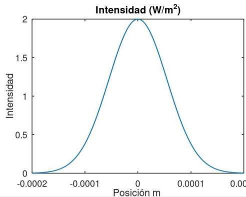
Figura 1: Perfil de Intensidad Gaussiano de la fuente láser
