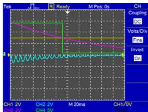
Figura 10. Señales de la unidad de sobrecorriente en condiciones de restablecimiento
