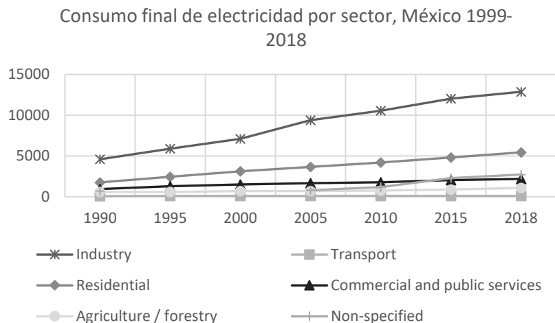
Figura 3. Grafica del consumo de electricidad por sectores
