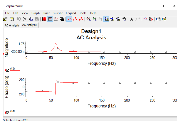
Figura 3. Respuesta del filtro pasabanda
