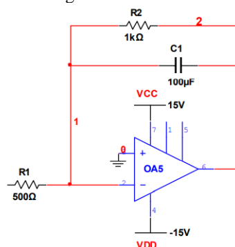
Figura 6. Circuito integrador
