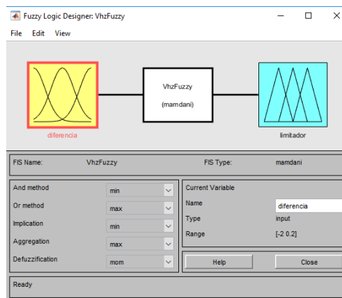
Figura 5. Toolbox para el diseño de lógica difusa.
