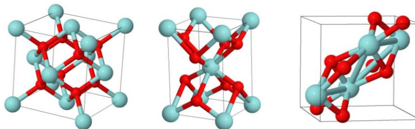
Figura 1.- Representación de la estructura cúbica, tetragonal y monoclinica de ZrO 2 .
