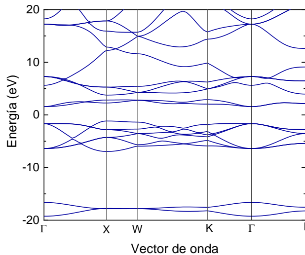
Figura 2.- Estructura de bandas electrónicas para la celda de ZrO 2 cúbica.
