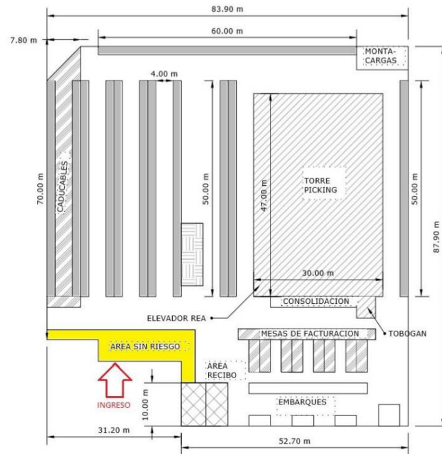
Imagen 1. Layout del almacén del centro de cumplimiento
