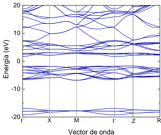
Figura 3.- Estructura de bandas electrónicas para la celda de ZrO 2 tetragonal.
