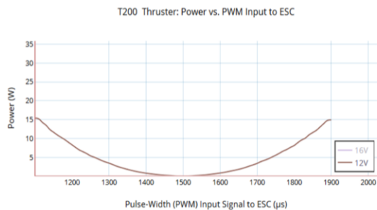
Figura 3. Características de los propulsores
