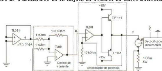
Figura 4. Etapa de potencia basada en el control de corriente.
