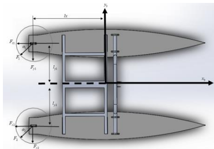
Figura 2. Actuadores azimutales.
