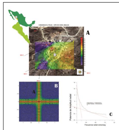
Figura 4. Comunidad del Frijol: (A) variación del campo magnético; (B) espectro de potencia de una celda reducida y (C) espectro de potencia radial con pendientes para profundidad de la discontinuidad de Mohorovich.
