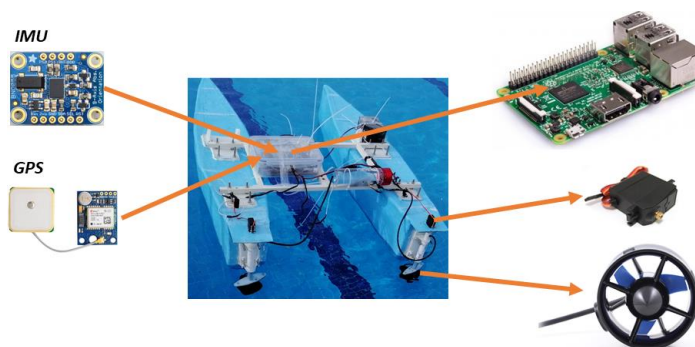
Figura 7. Sensores y actuadores del USV.
