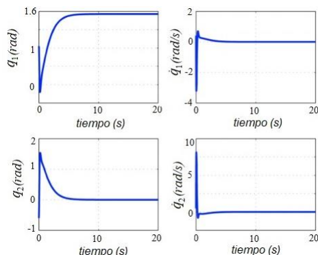
Figura 6. Estabilización de estados mediante simulación
