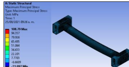
Figura 6 Máximo estrés principal rodillo
