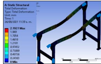
Figura 11 Deformación total módulo
