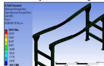
Figura 12 Máximo estrés principal módulo
