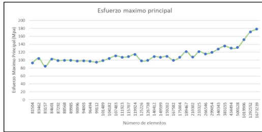
Gráfica 3 Comportamiento de esfuerzo máximo
