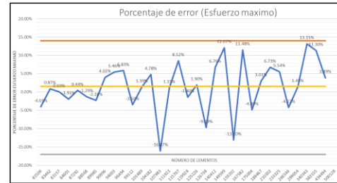
Gráfica 4 Porcentaje de error de esfuerzo máximo
