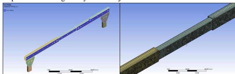
Figura 3 Parametrización de mallado lateral
