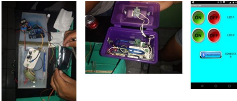
Ilustración 7 Conexión Arduino uno, Arduino nano y servomotores; Conexión Arduino nano y Bluetooth y Accionamiento vía Bluetooth
