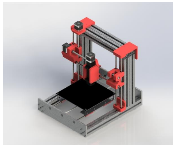
Figura 2. Diseño de la primera etapa de la impresora – Modo CNC
